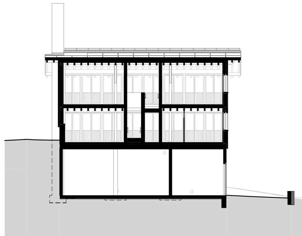
GEBÄUDESCHNITT 1
