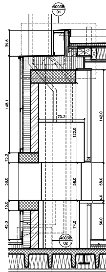
05 COUPE FACADE EST (BLOC CHEMINEE) 1:20
