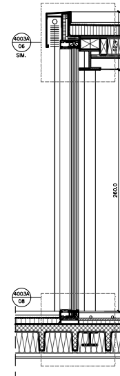
06 COUPE FACADE EST (TERRASSE) 1:20
