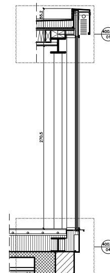
04 COUPE FACADE EST (TOITURE VEG.) 1:20
