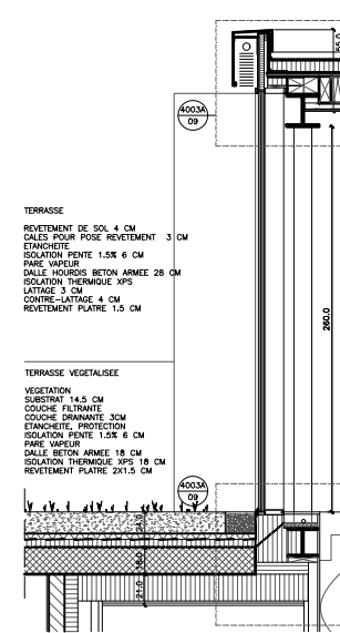
04 COUPE FACADE EST (TOITURE VEG.) 1:20
