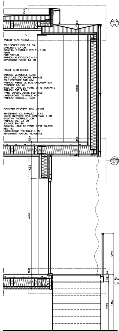
03 COUPE FACADE OUEST (BLOC CUISINE) 1:20
