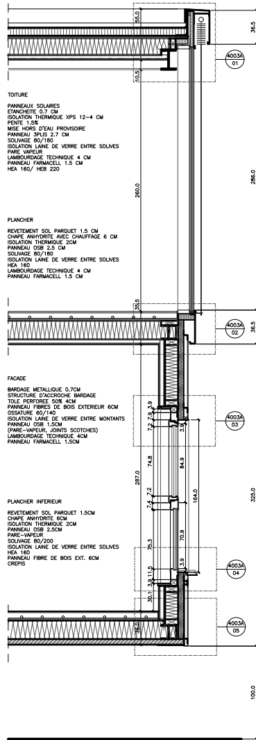
01 COUPE FACADE NORT 1:20
