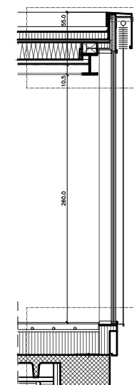
08 COUPE FACADE OUEST (PORTE COULISSANTE) 1:20
