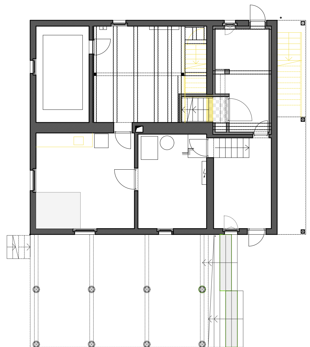
Untergeschoss 1:100
