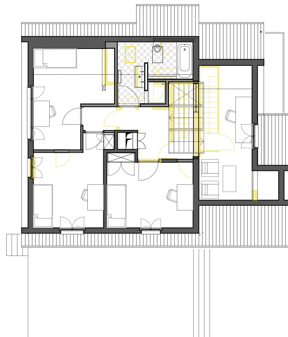
Obergeschoss 1:100
