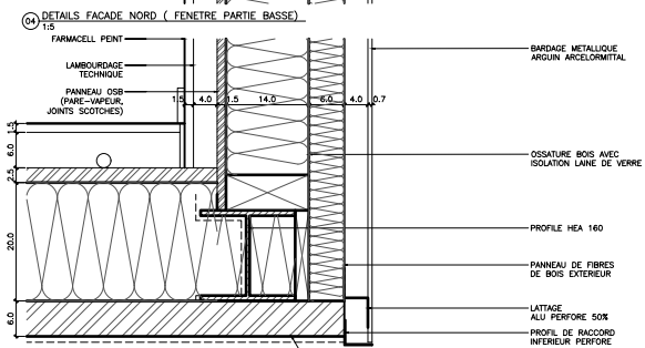
13 DETAILS FACADE NORD (PORTE-A-FAUX) 1/5
