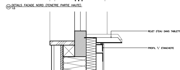
10 DETAILS FACADE NORD ( FENÊTRE PARTIE BASSE) 1/5
