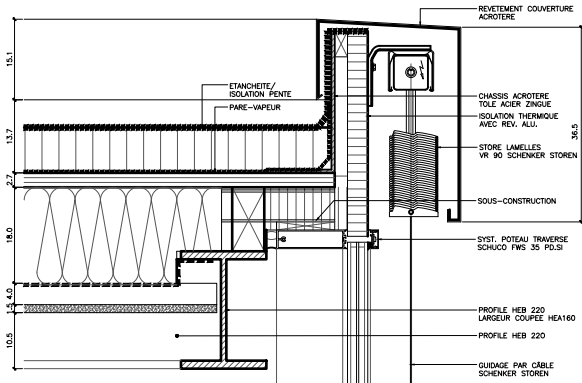
01 DETAILS FACADE NORD ACROTÈRE 1/5
