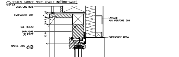
07 DETAILS FACADE NORD (FENÊTRE PARTIE HAUTE) 1/5
