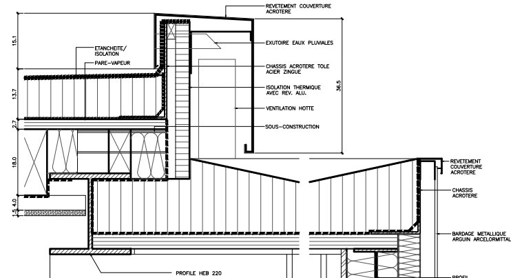
03 DETAILS FACADE OUEST (TOITURE BLOC CUISINE) 1/5
