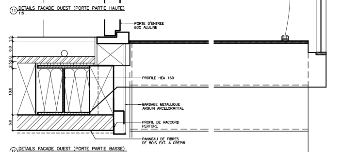
12 DETAILS FACADE OUEST (PORTE PARTIE BASSE) 1/5
