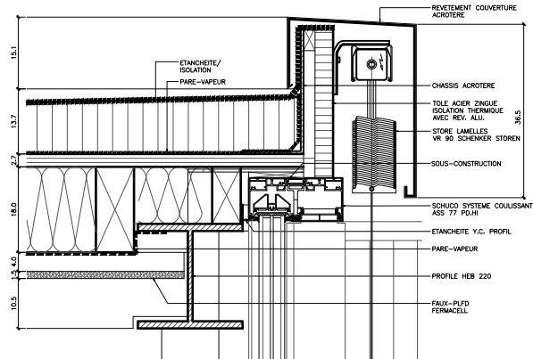
02 DETAILS FACADE OUEST ( ACROTÈRE, FENÊTRE COULISSANTE) 1/5
