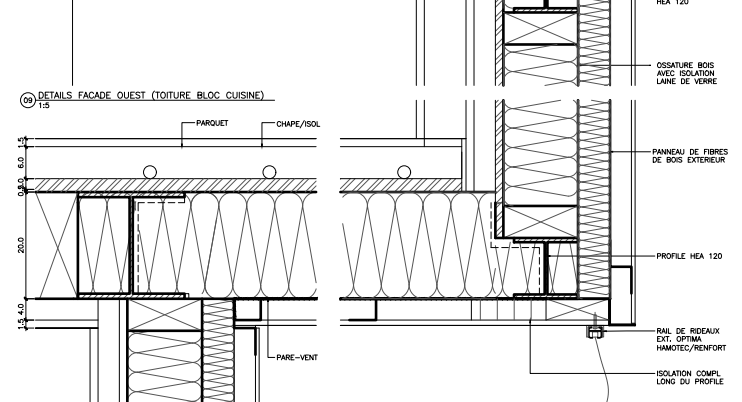
06 DETAILS FACADE OUEST (DALLE BLOC CUISINE) 1/5
