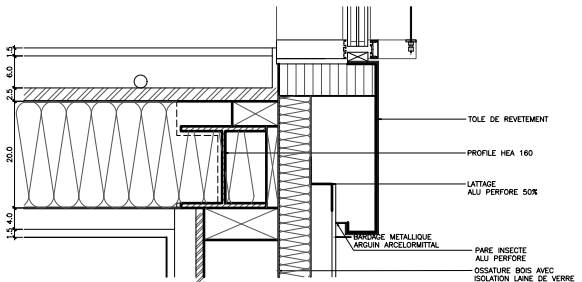
04 DETAILS FACADE NORD (DALLE INTERMEDIAIRE) 1/5
