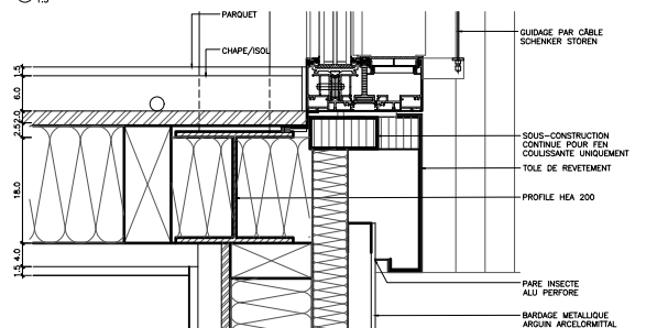
05 DETAILS FACADE OUEST ( FENÊTRE COULISSANTE) 1/5
