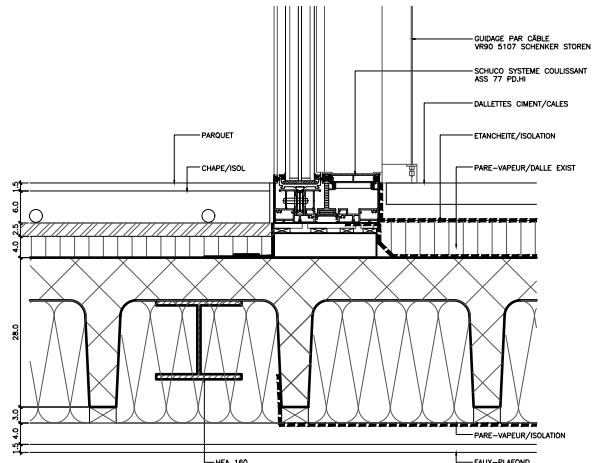
11 DETAILS FACADE EST ( FENÊTRE COULISSANTE) 1/5
