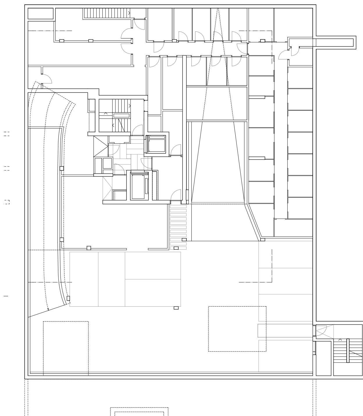
1. UG Zeichnungsmaßstab 1:200
