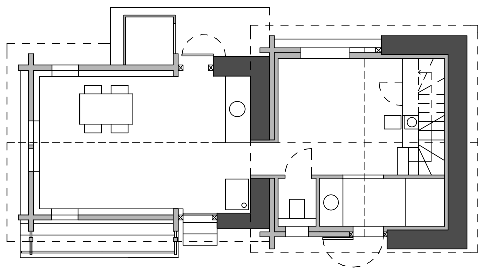
rez-de-chaussée
