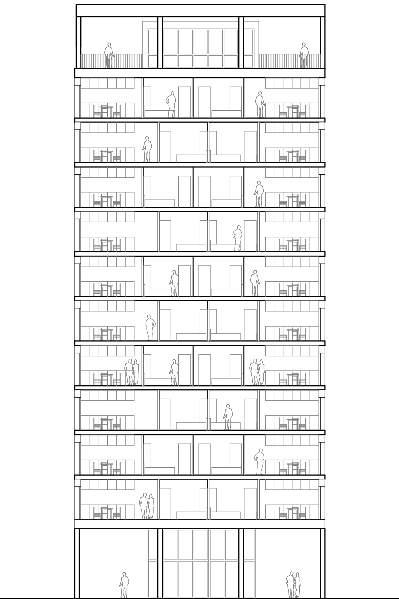
1/1000 [COUPE A-A]
