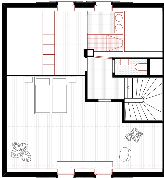
Dachgeschoss 1:100
