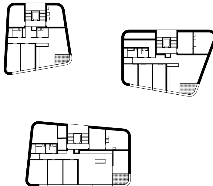
Grundriss EG
