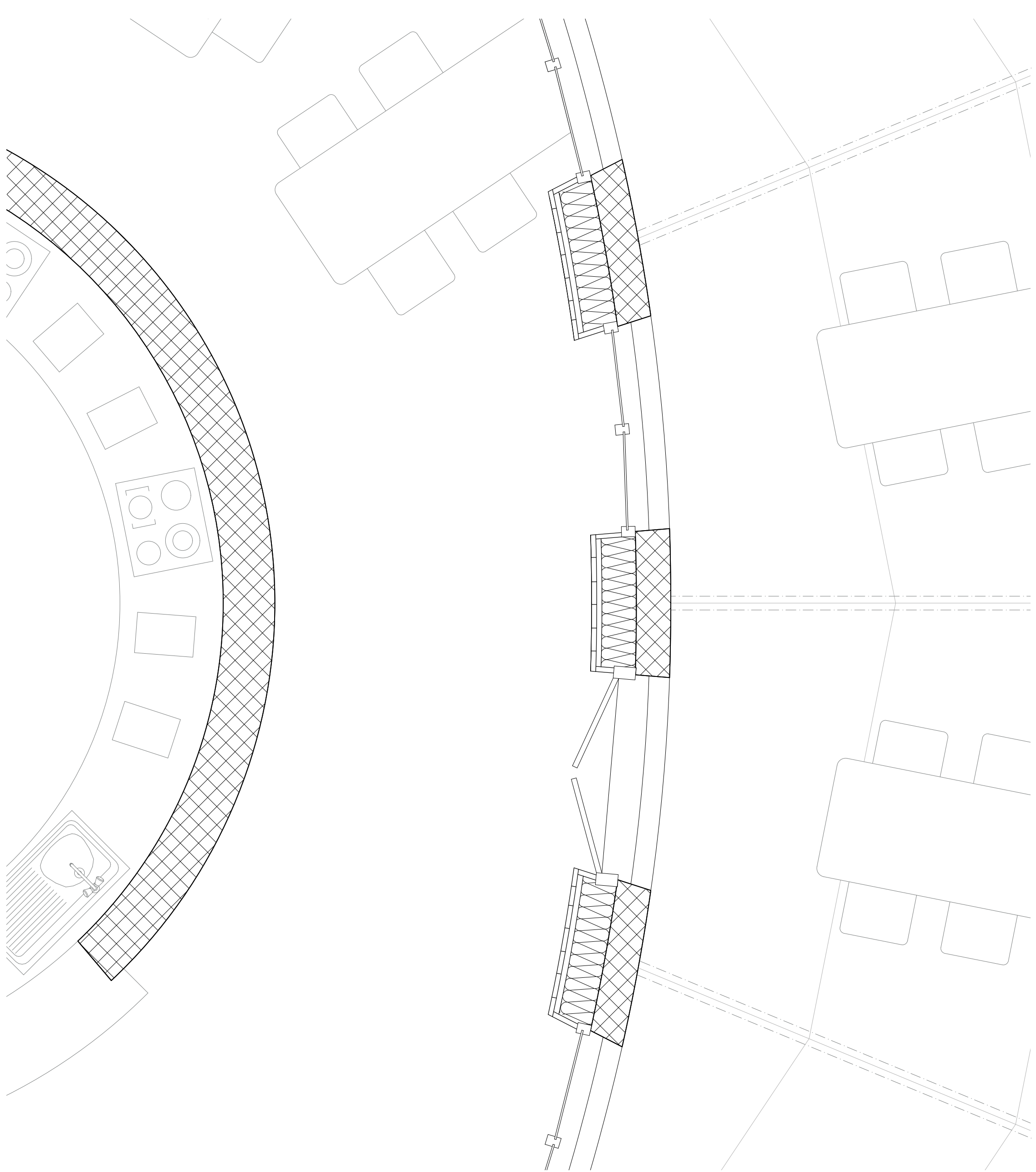
Grundrissausschnitt 1:20
