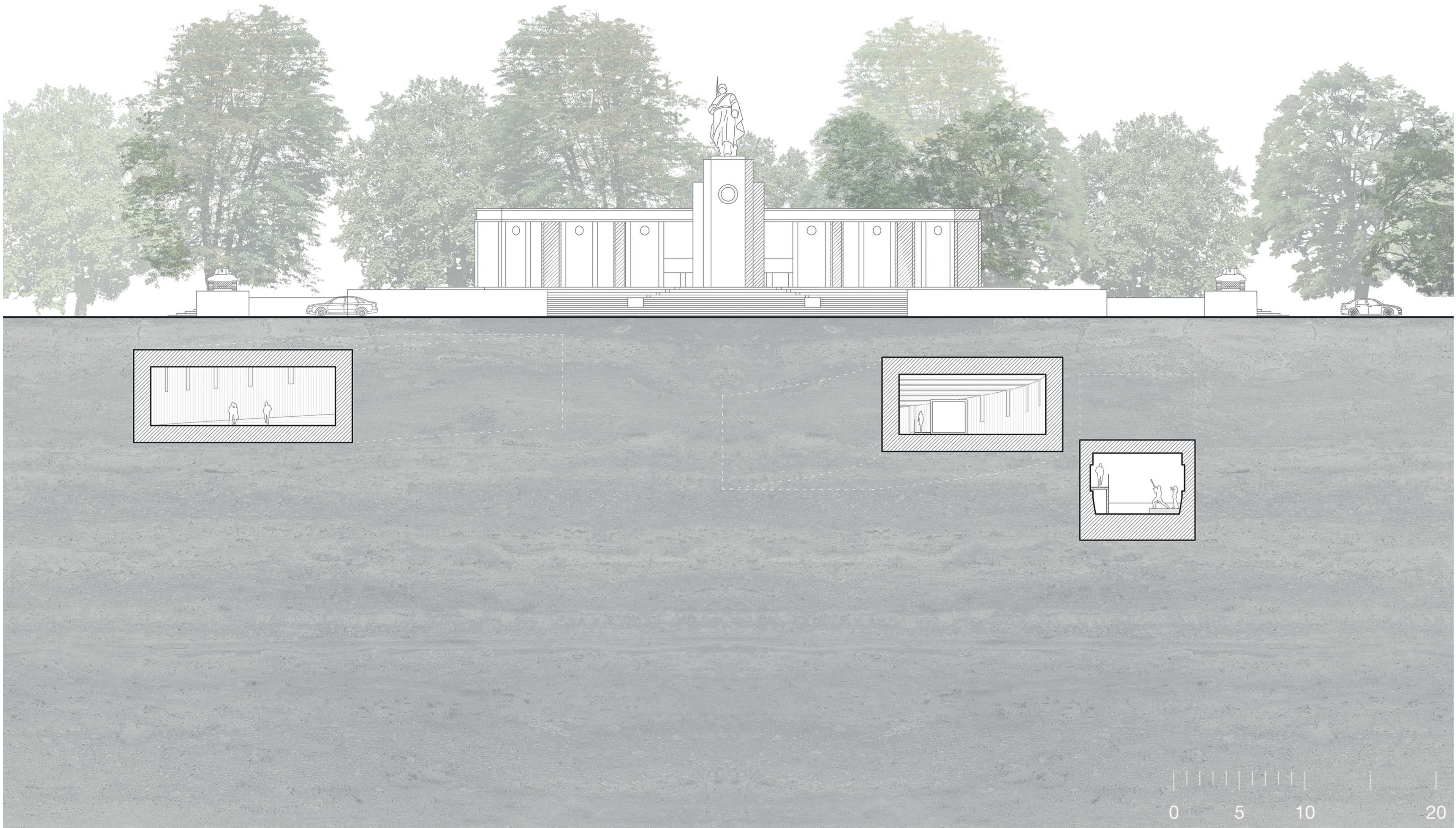
COUPE G-G 1:200
