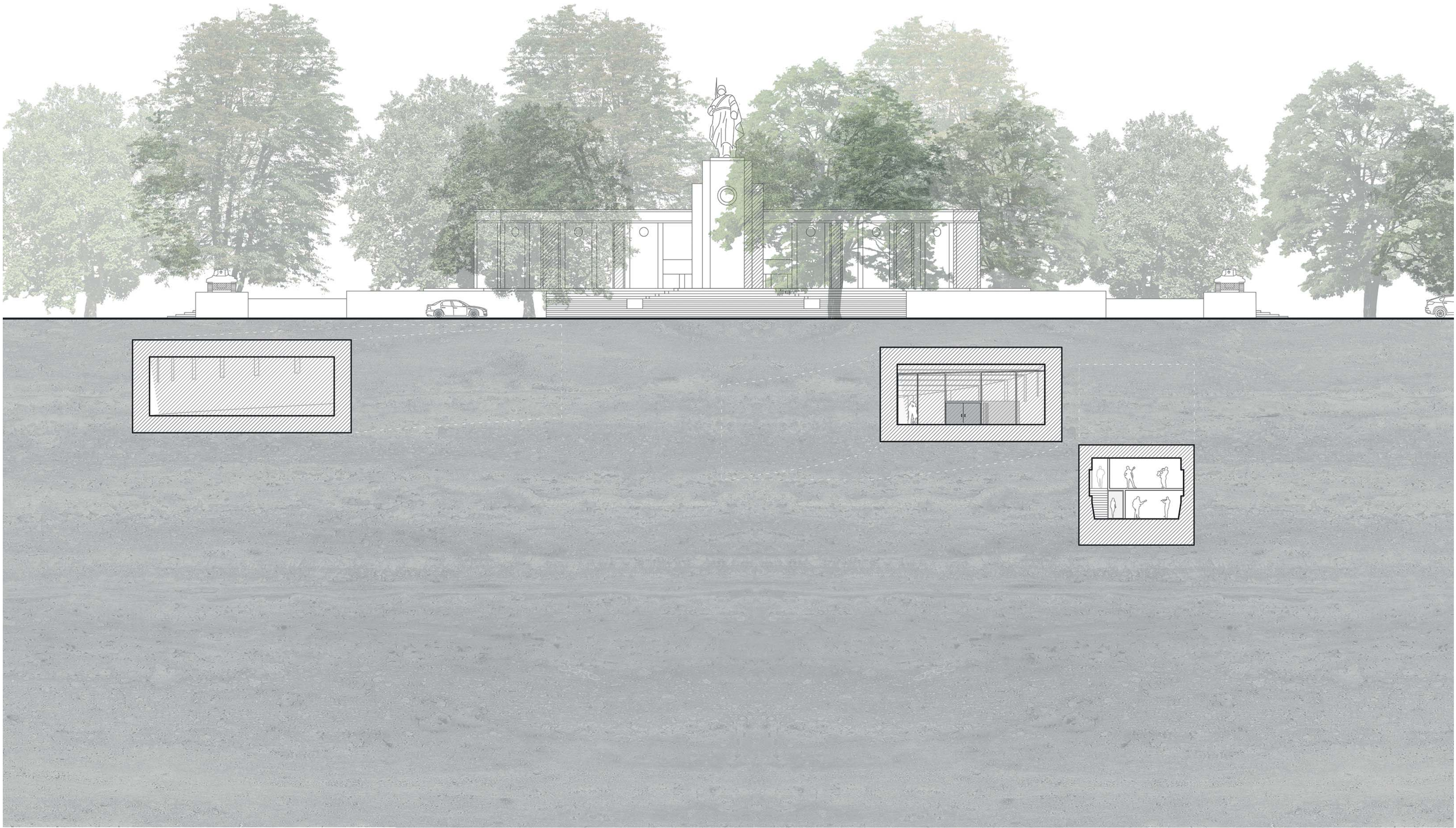
COUPE TRANSVERSALE F-F 1:200
