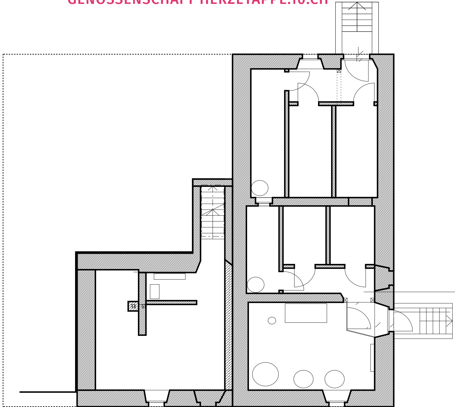
UNTERGESCHOSS
