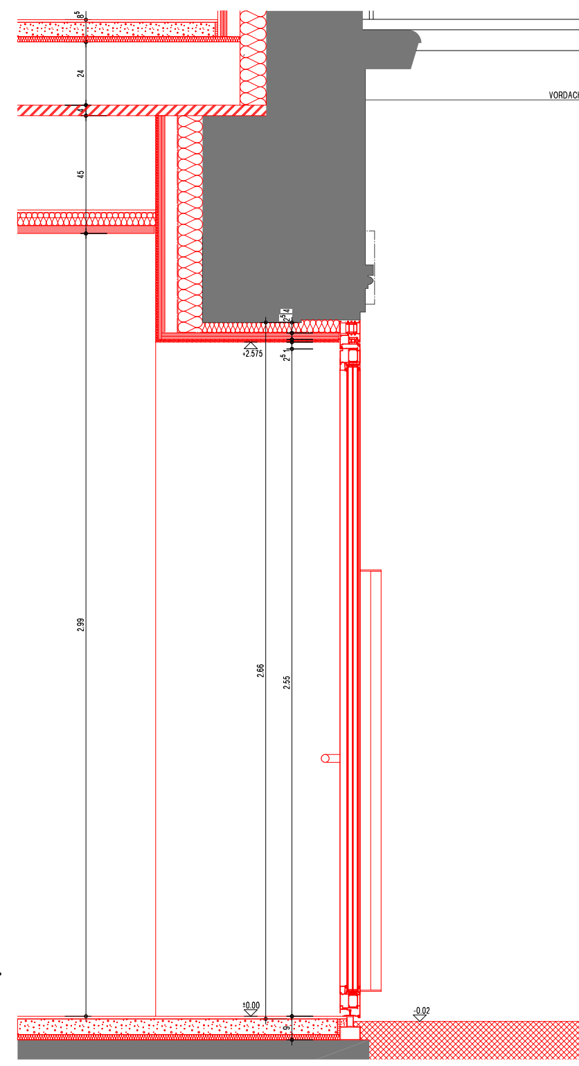
SCHNITT
