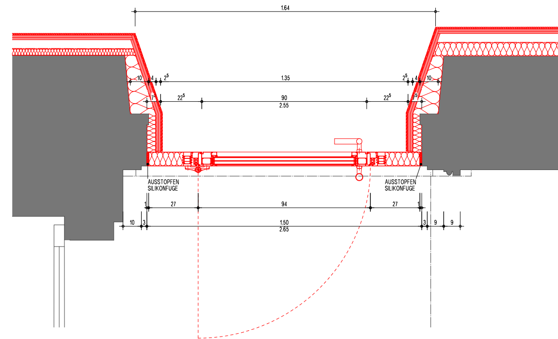
GRUNDRISS
