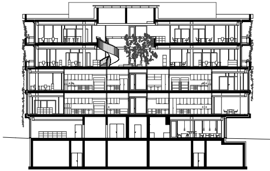
Schnitt A | Coupe A
