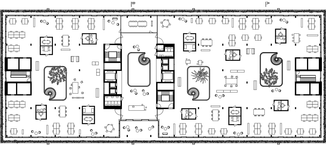
4. Obergeschoss | 4 ème étage
