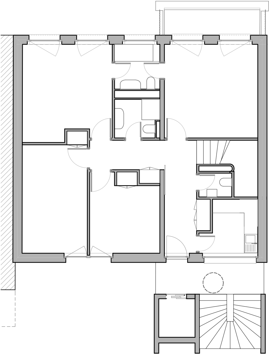
Etage 7
