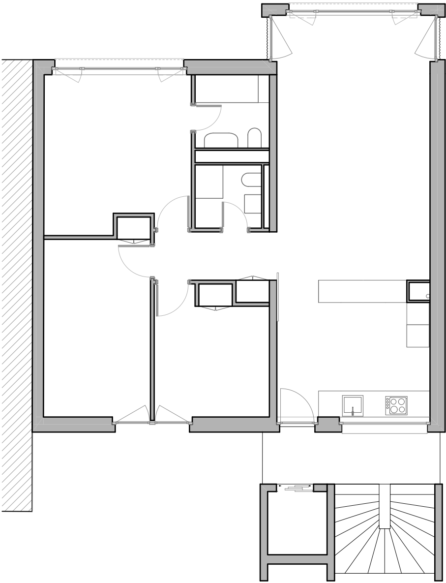
Etage type
