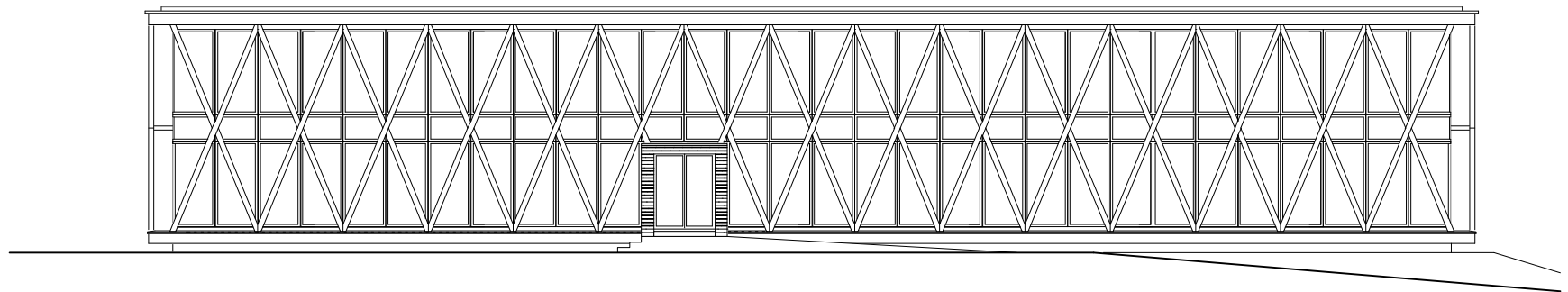
Nordfassade Mst. 1:200
