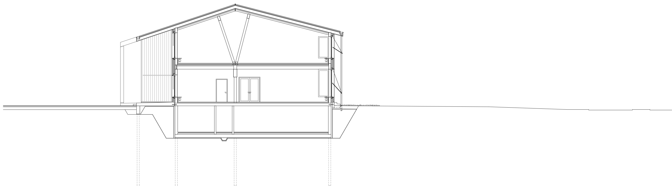
Schnitt
