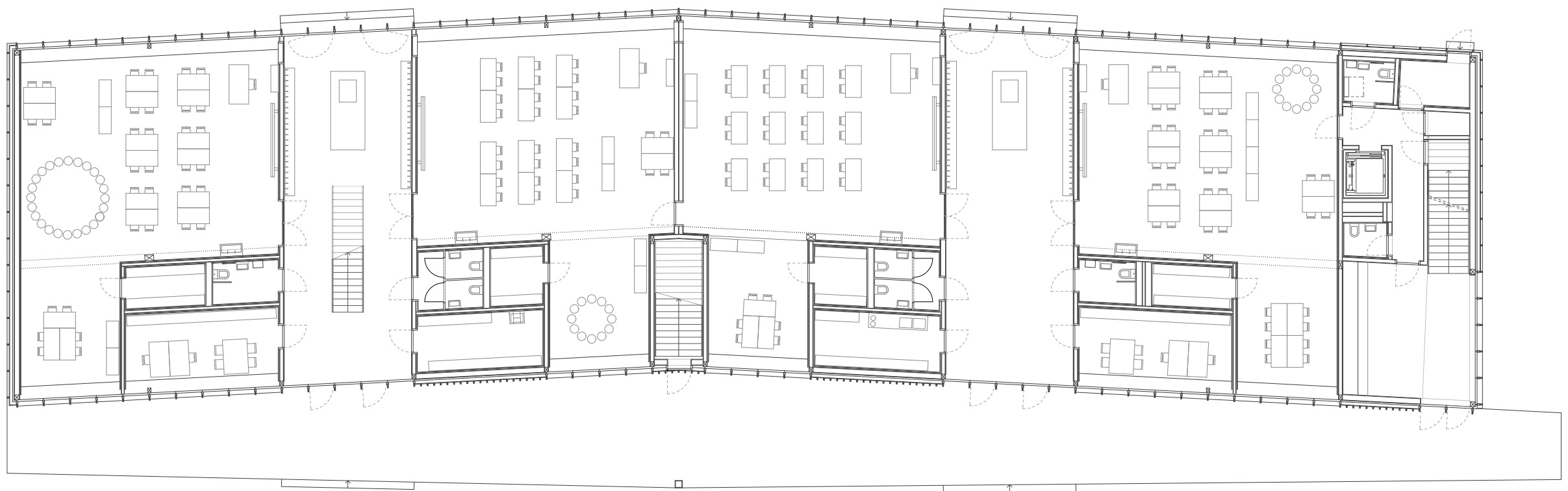
Erdgeschoss
