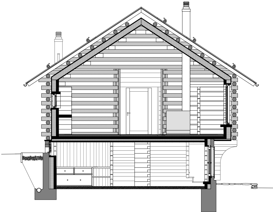
SCHNITT B - B
