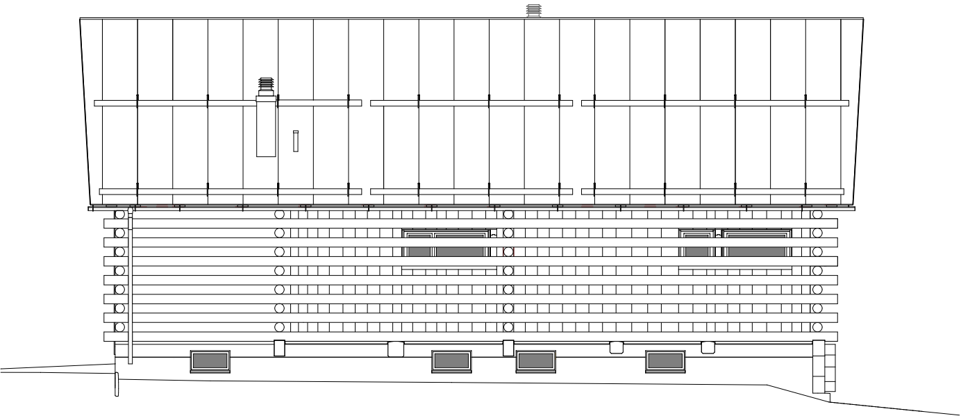
ANSICHT NORD - WEST
