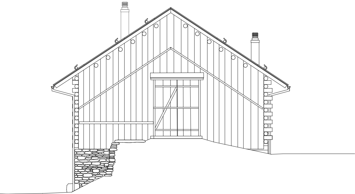
ANSICHT NORD - OST
