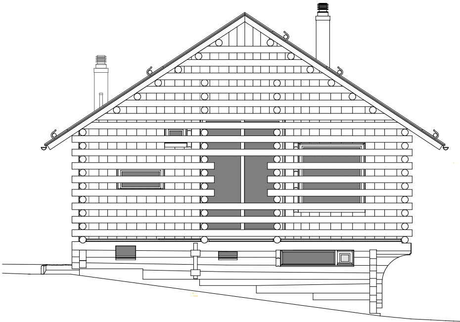
ANSICHT SÜD - WEST
