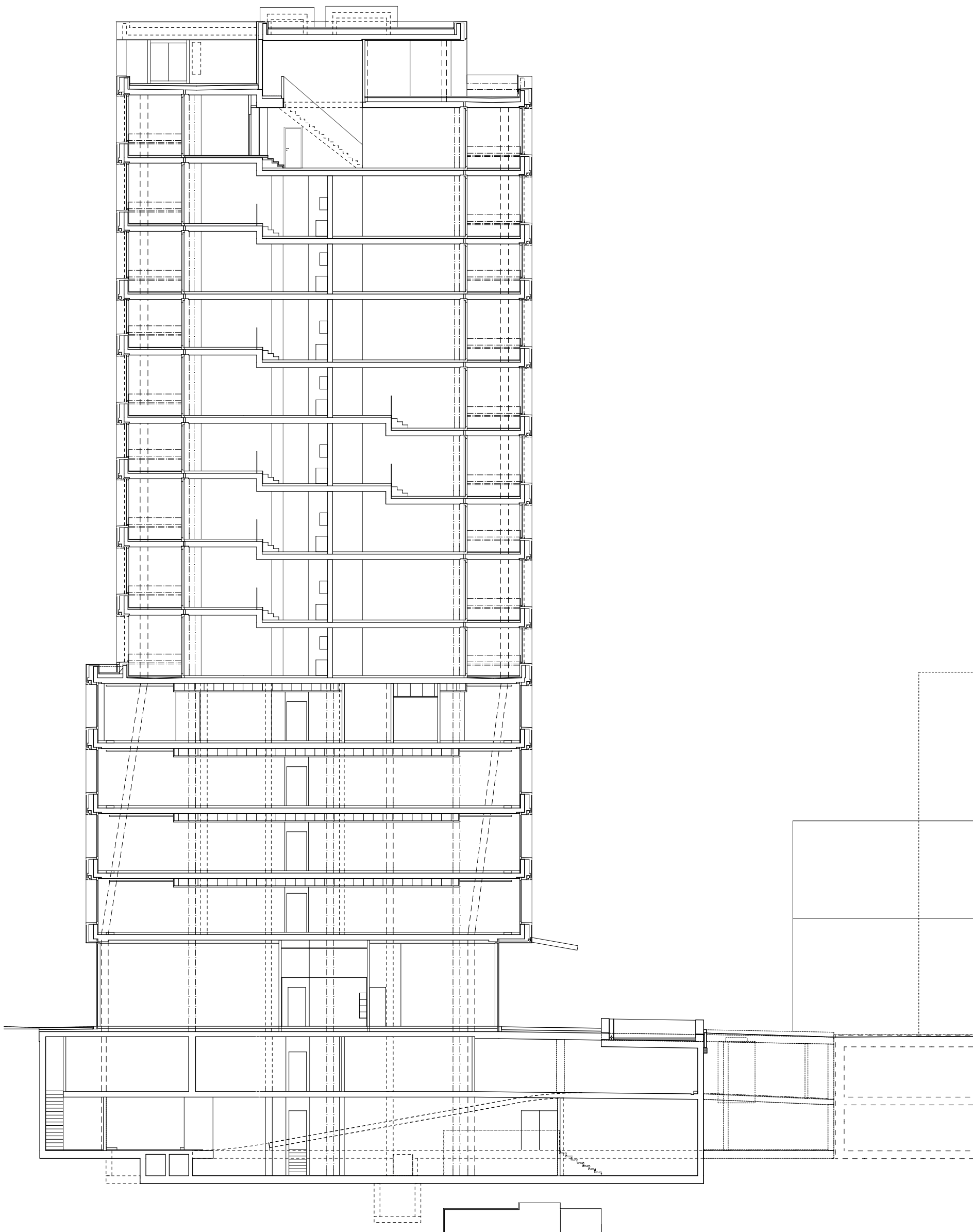
SCHNITT C1-C1 Zeichnungsmaßstab 1:200
