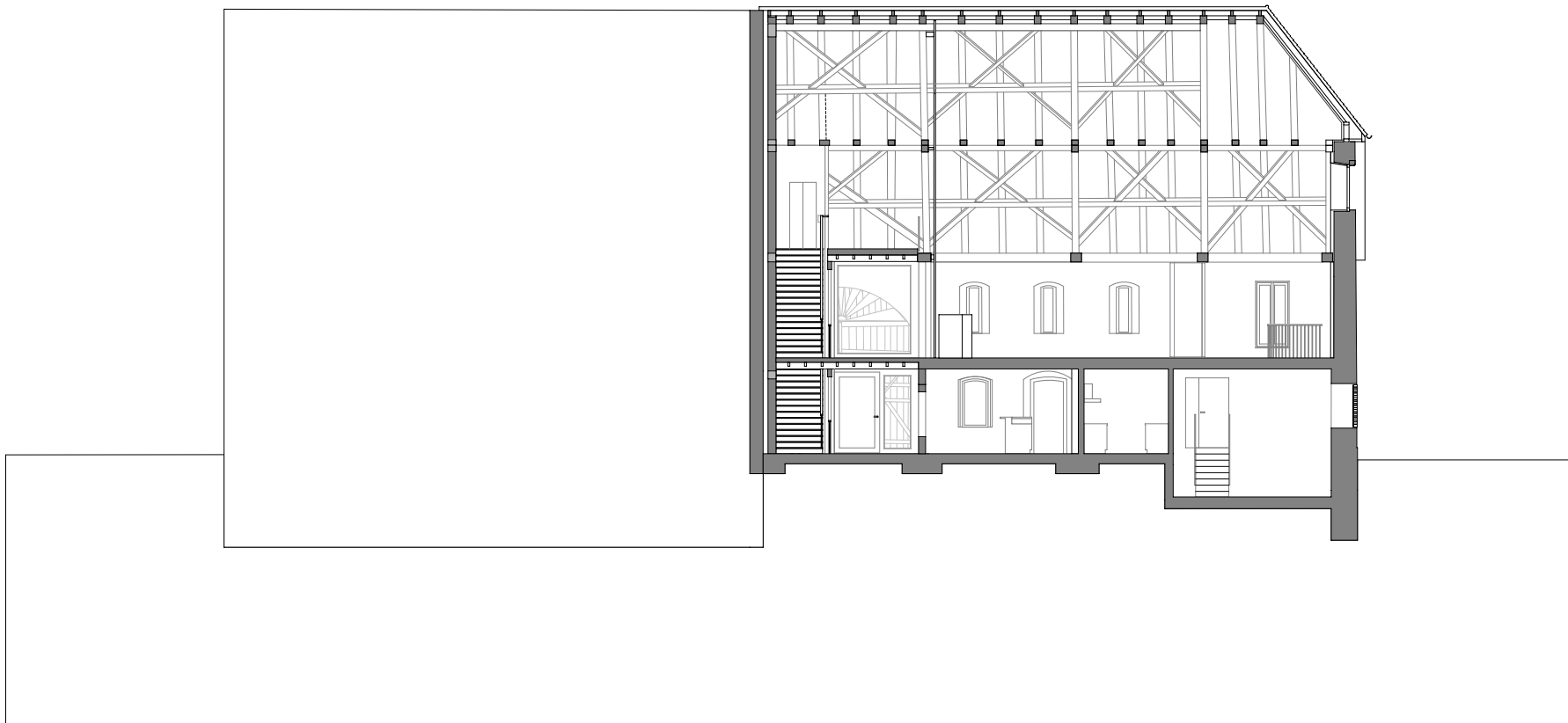
Längsschnitt 1:200
