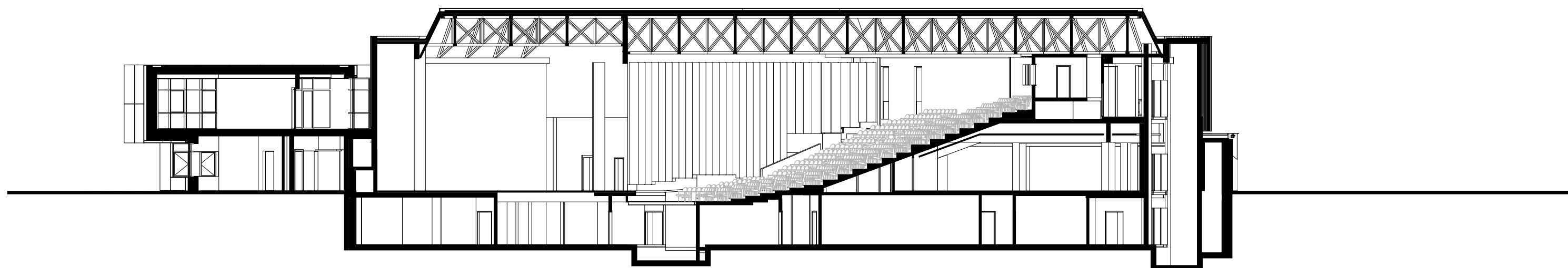
LONGITUDINALE
