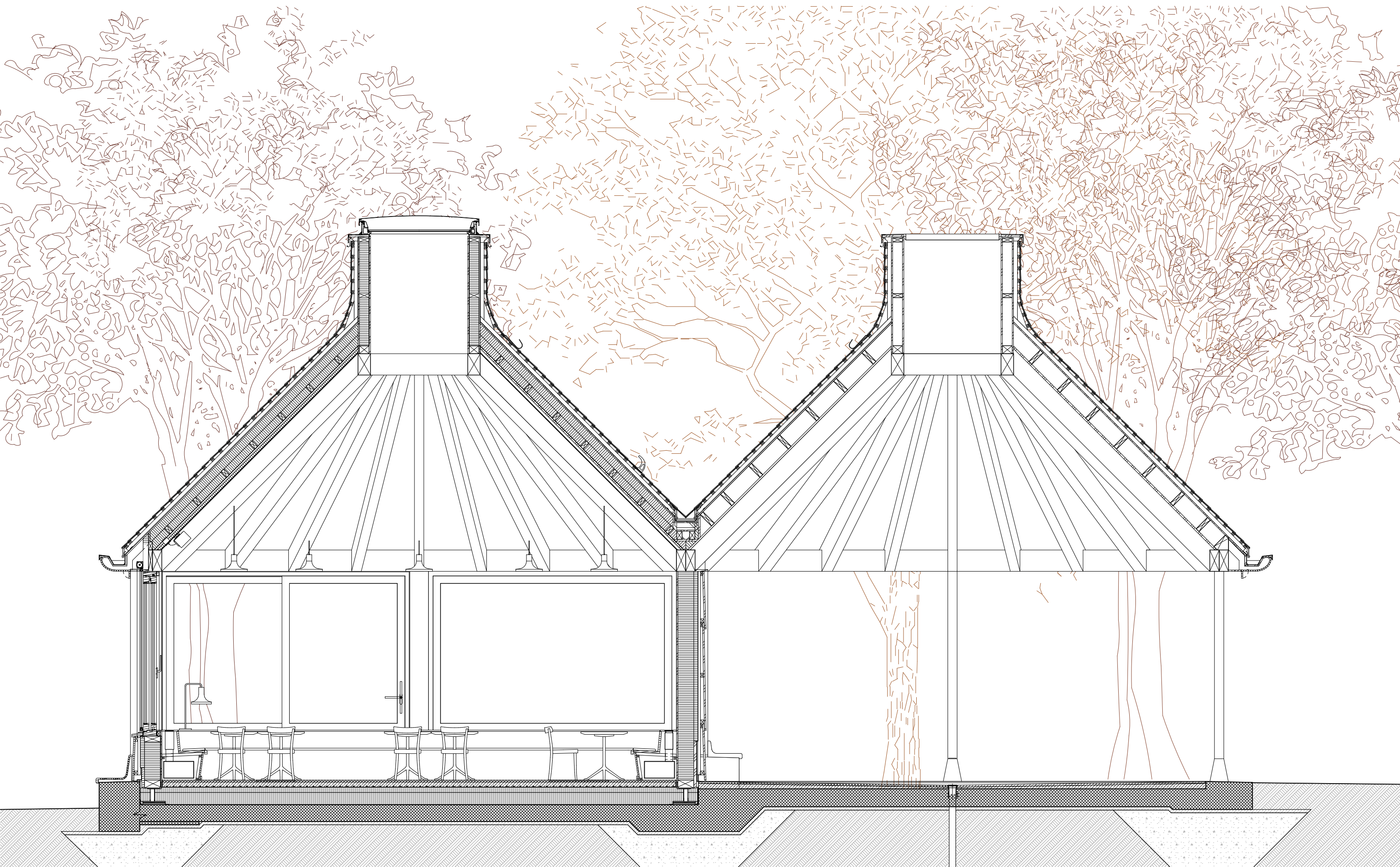
Konstruktionsschnitt 1:50
