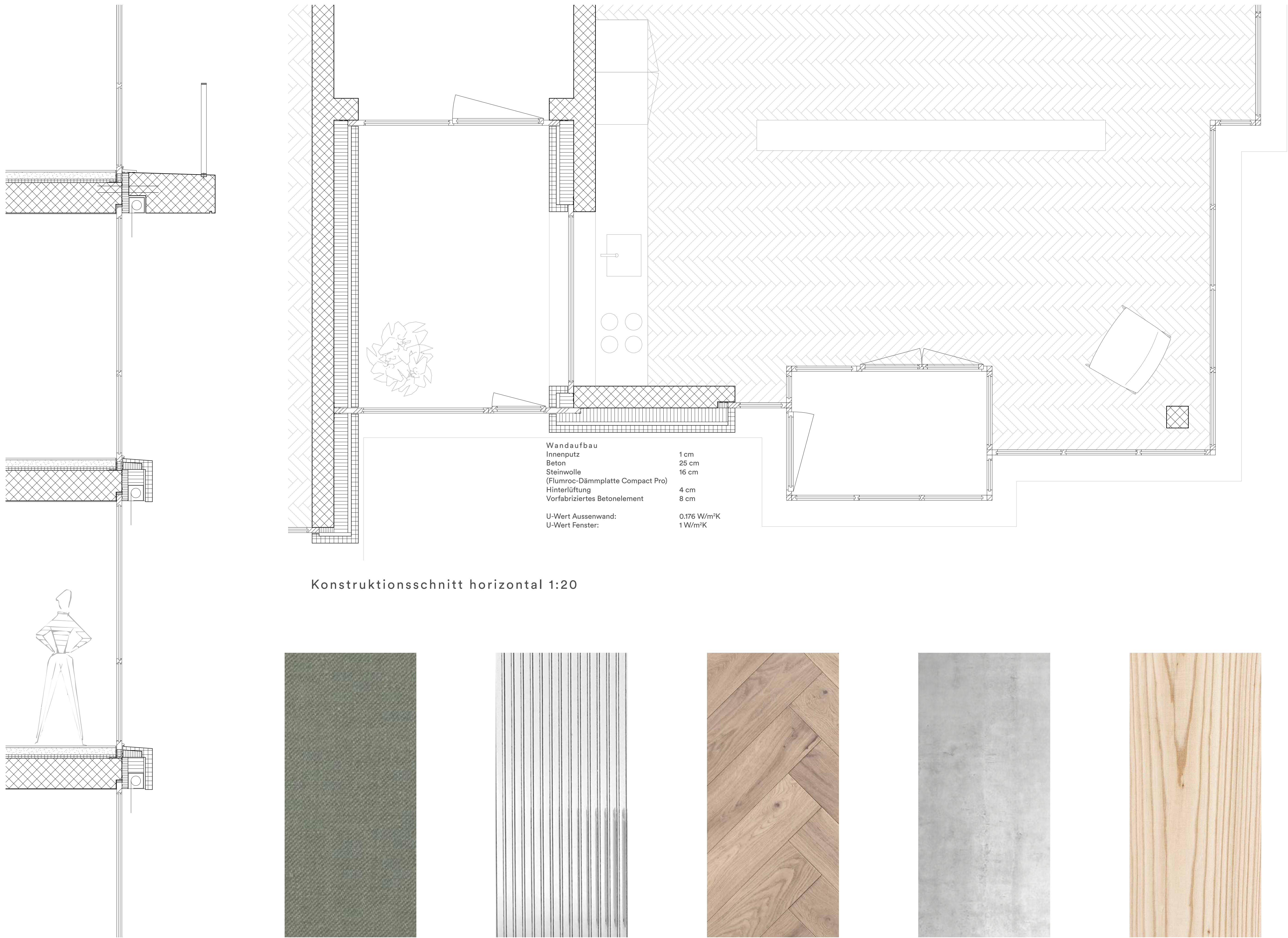
Konstruktionsschnitt vertikal 1:20
