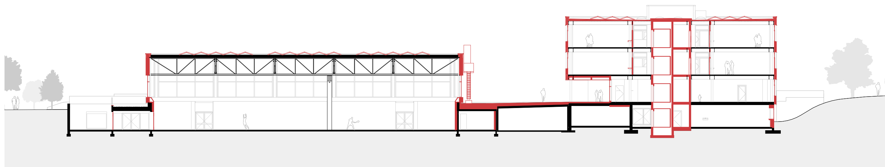
Coupe A - 1:300
