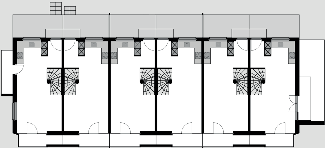
Grundriss Erdgeschoss
