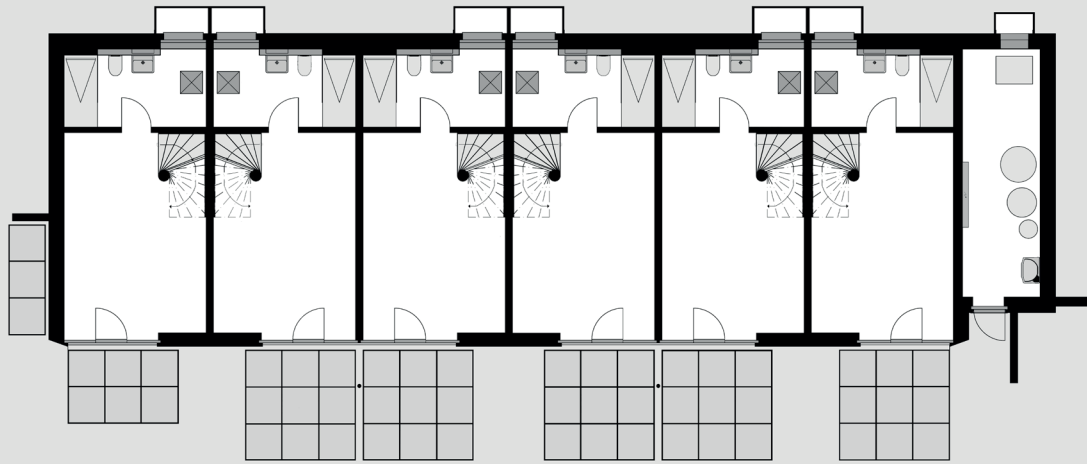
Grundriss Untergeschoss
