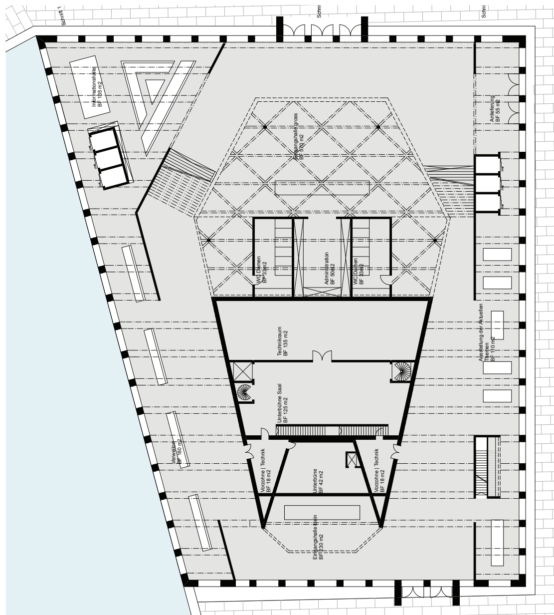
Erdgeschoss 1:400
