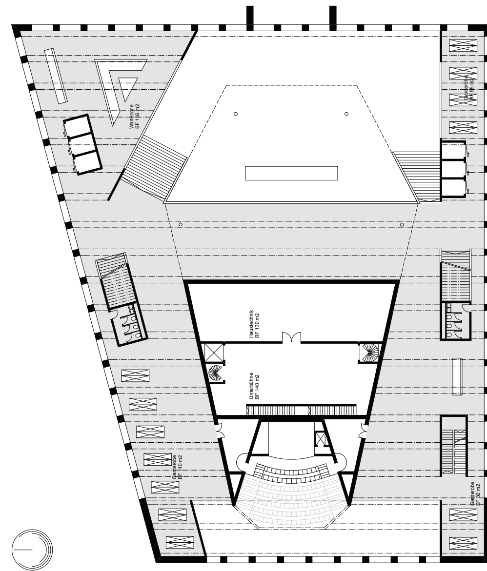
EG Zwischengeschoss 1:400
