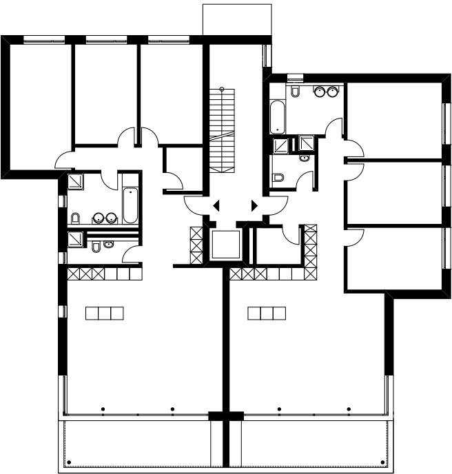
Normgeschoss
