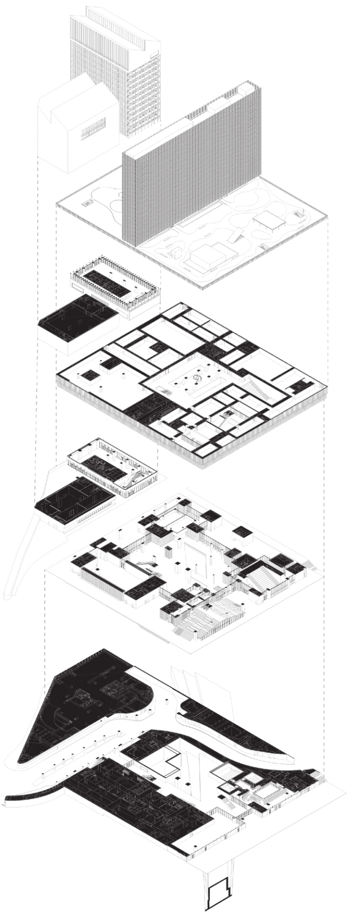
Explosionsaxonometrie | Explosion axonométrique
