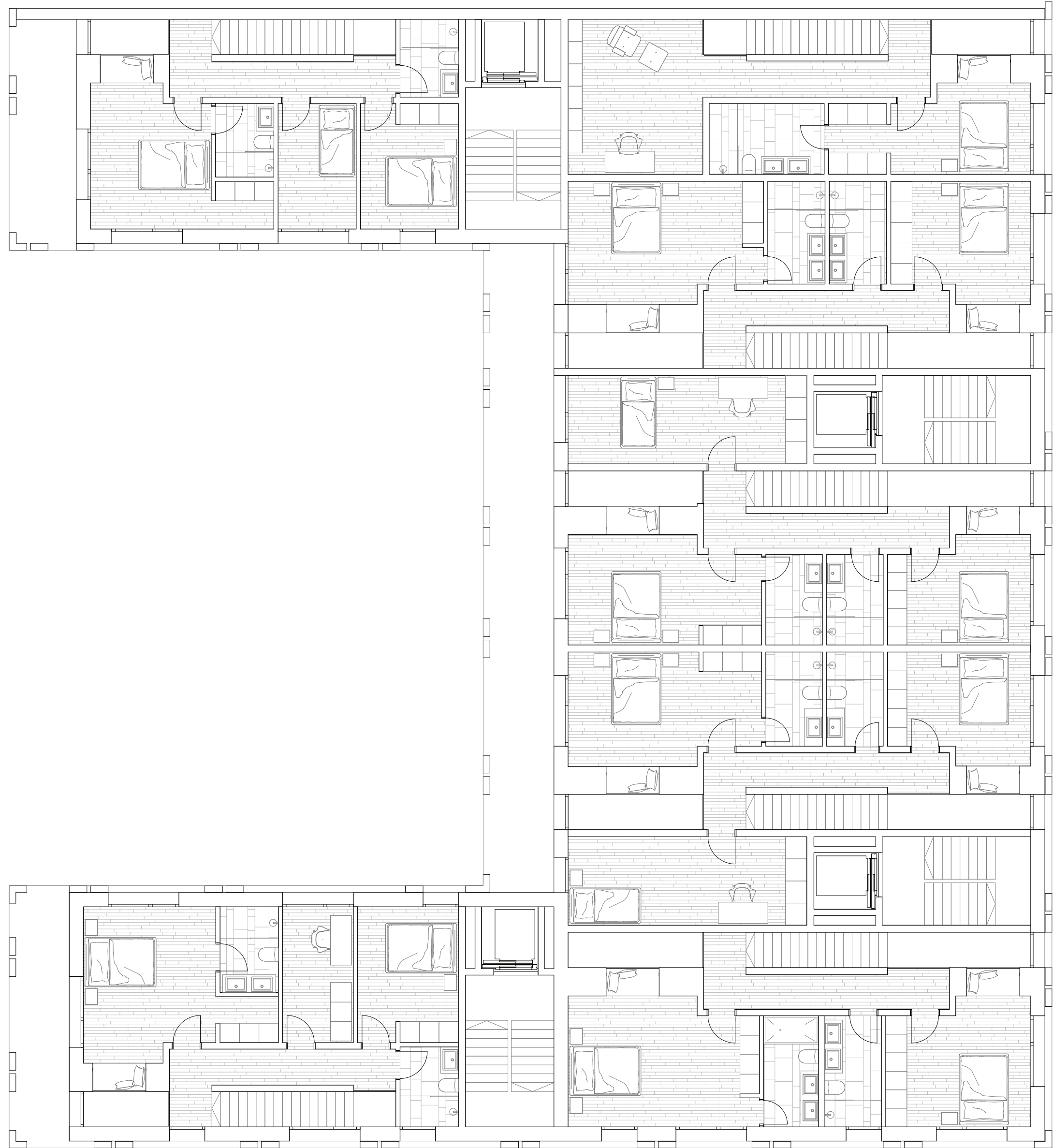
2. Obergeschoss M 1|100
