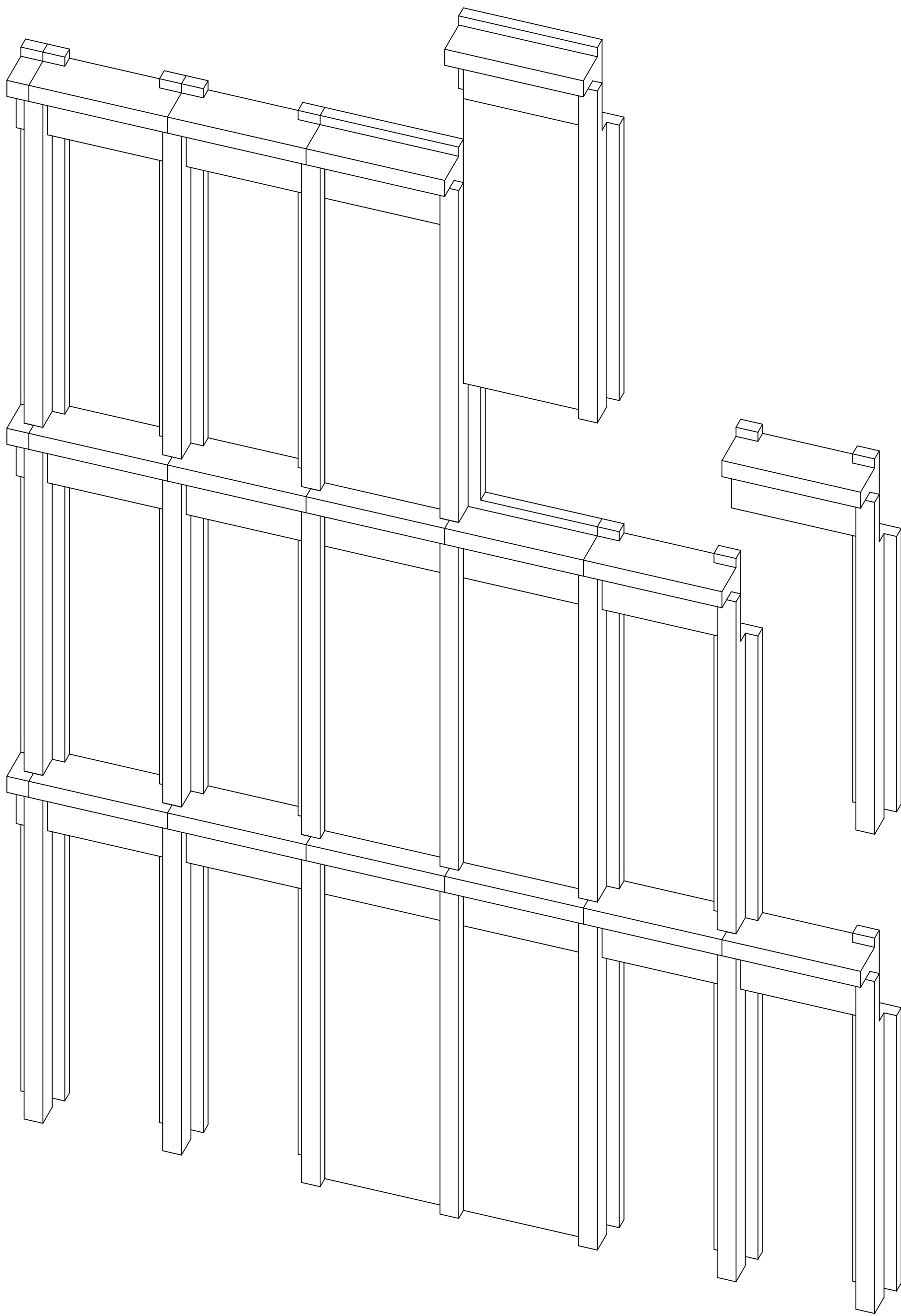
Axonometrie zum Fügungsprinzip der Fassadenelemente
