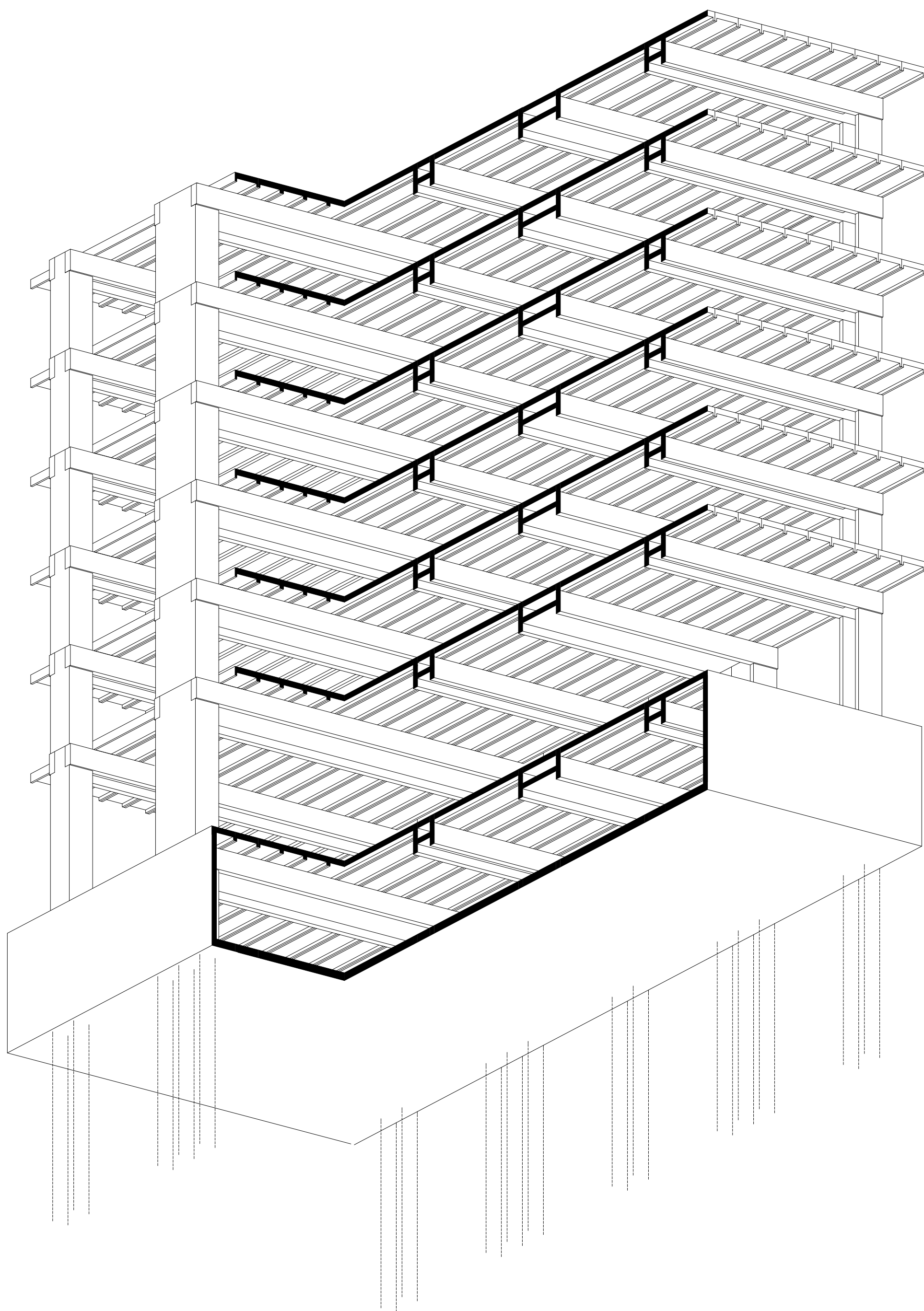
Tragwerks-Axonometrie
