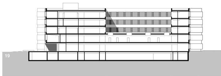
Schnitt B
