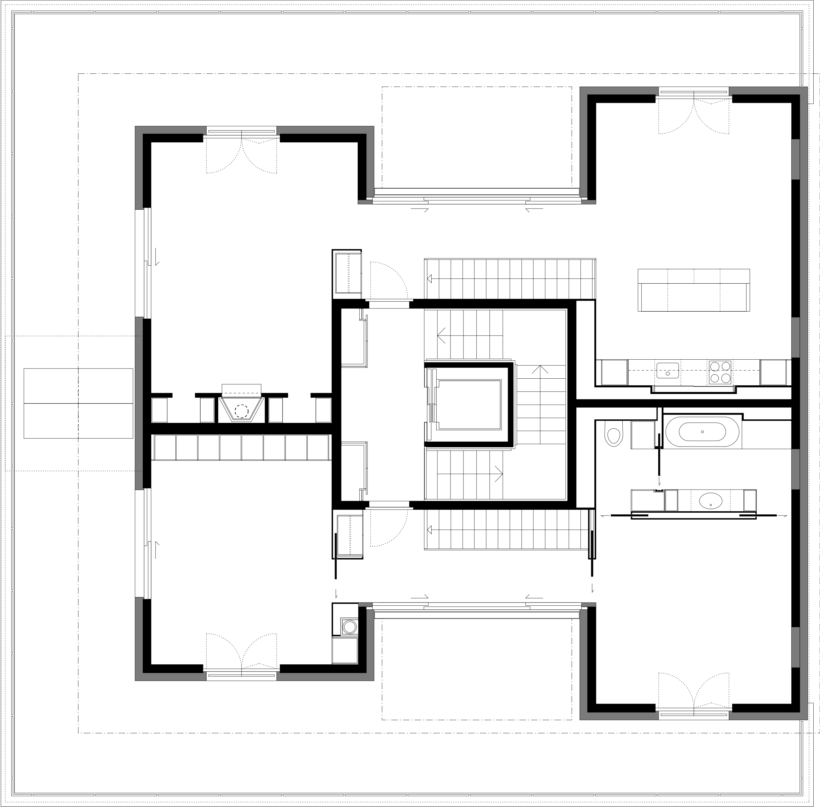
7. OG - ATTIKA
