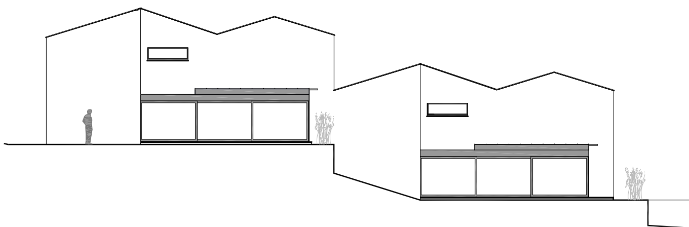
FACADE OUEST
