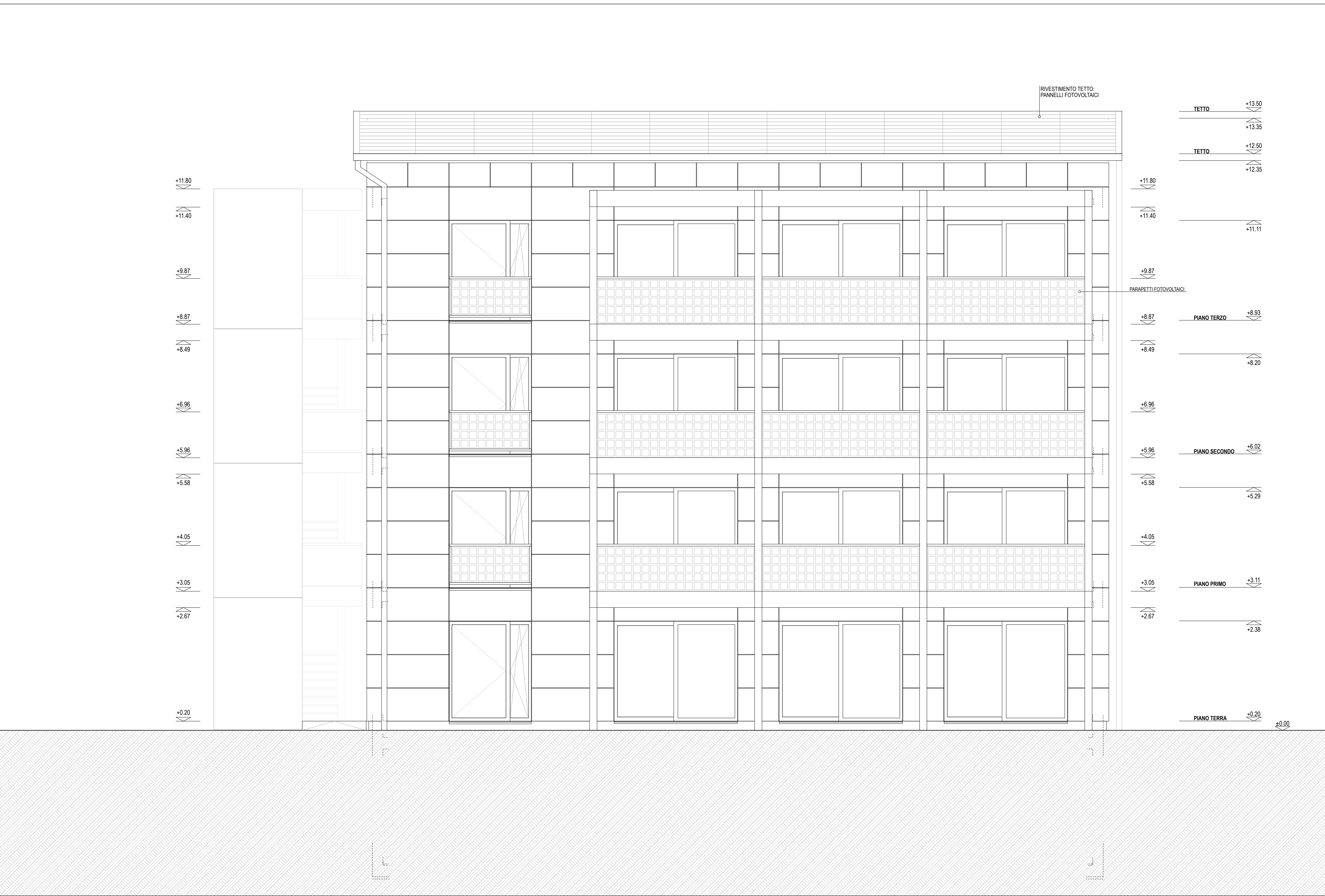
FACCIATA SUD-OVEST | SCALA 1:50
