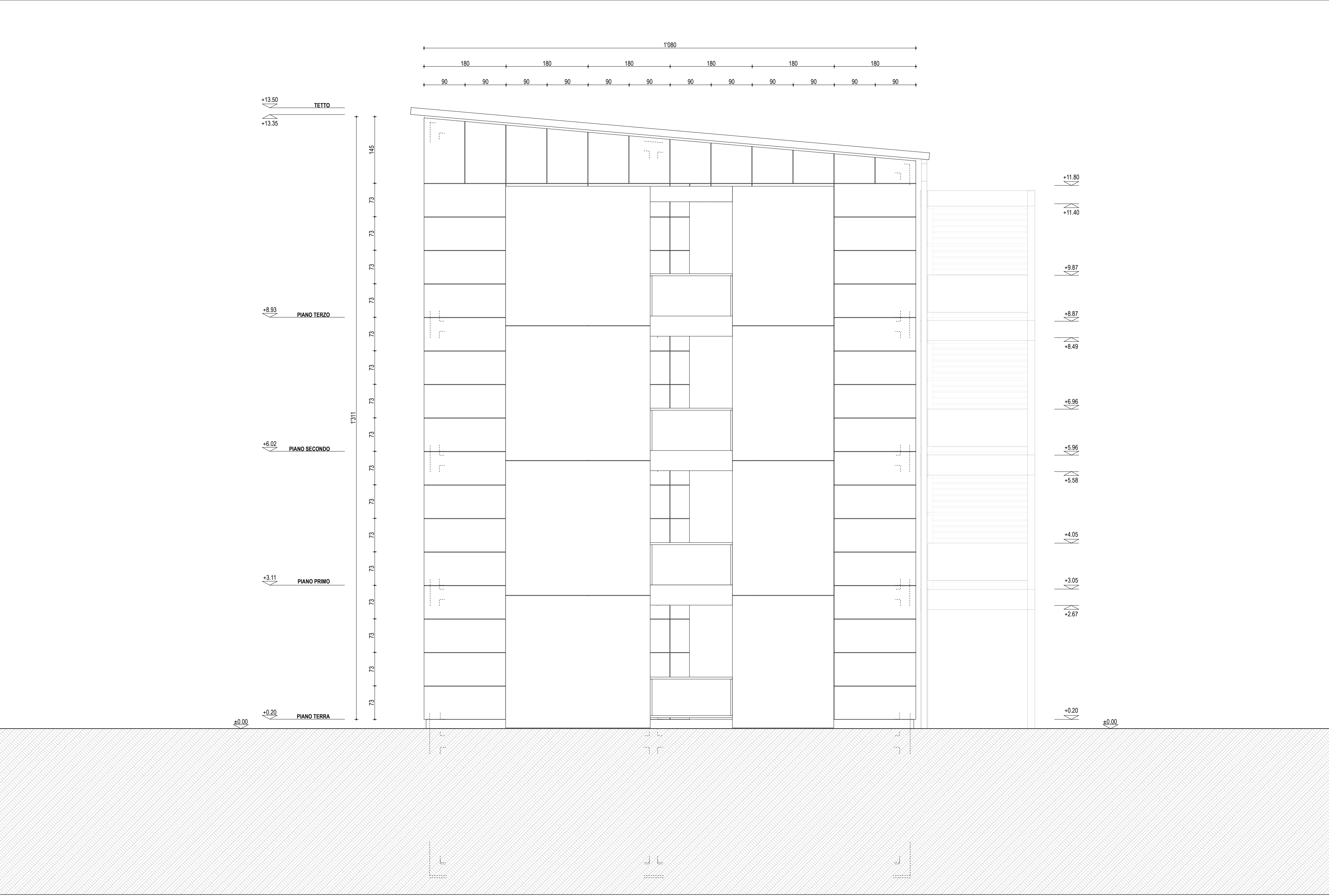
FACCIATA NORD-OVEST | SCALA 1:50
