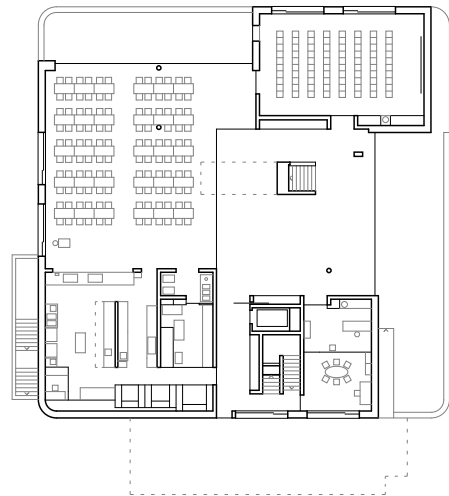
rez-de-chaussée
