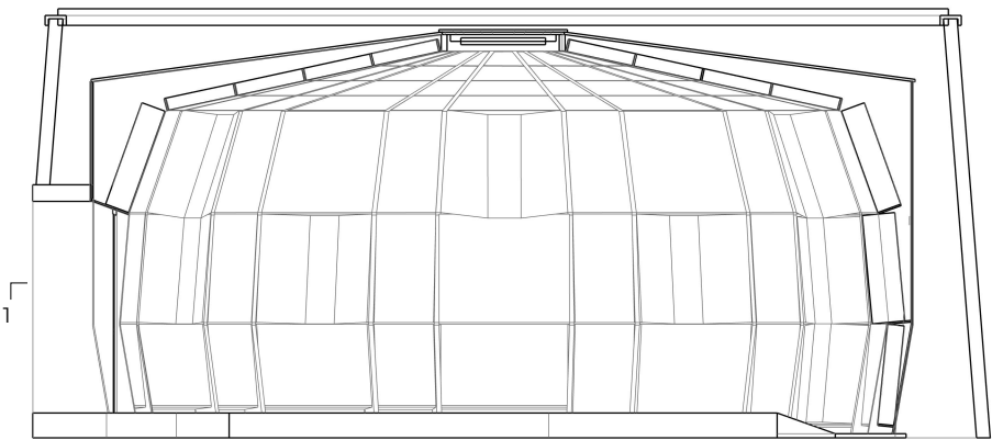
Schnitt A-A
