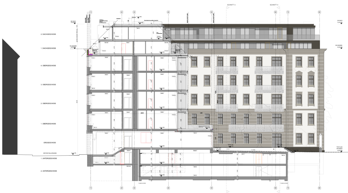
Querschnitt
