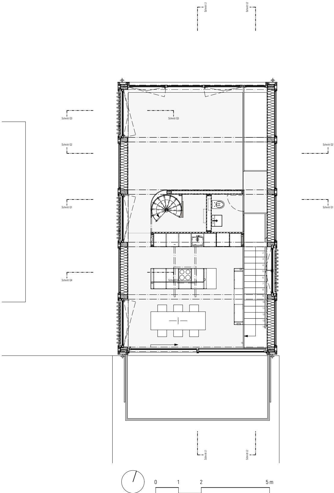
Ausführung 2.OG 1:100
