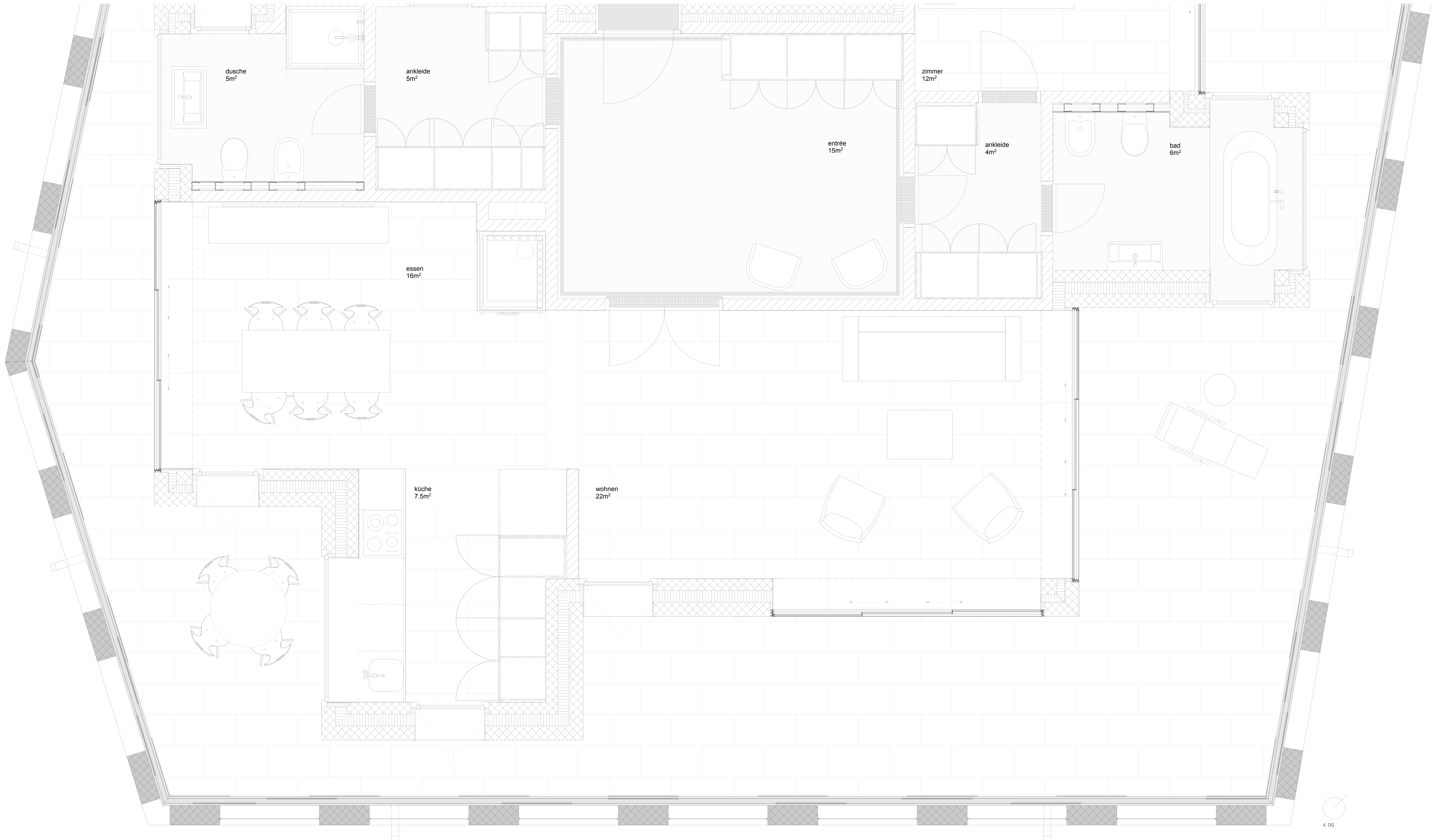
Grundriss 1:20
