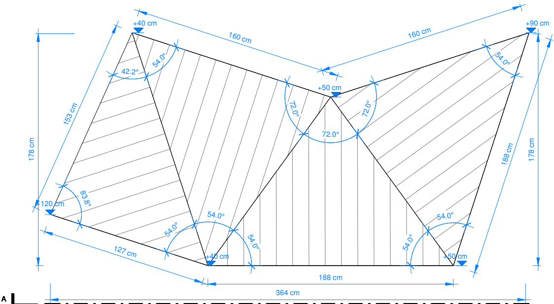
Grundriss 1 : 20
