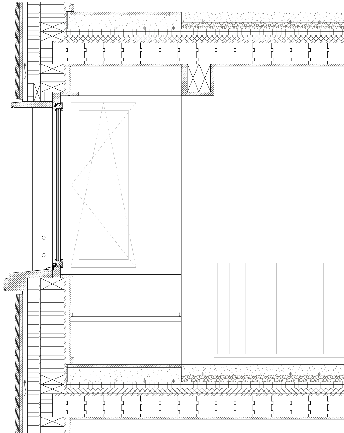
Schnitt
