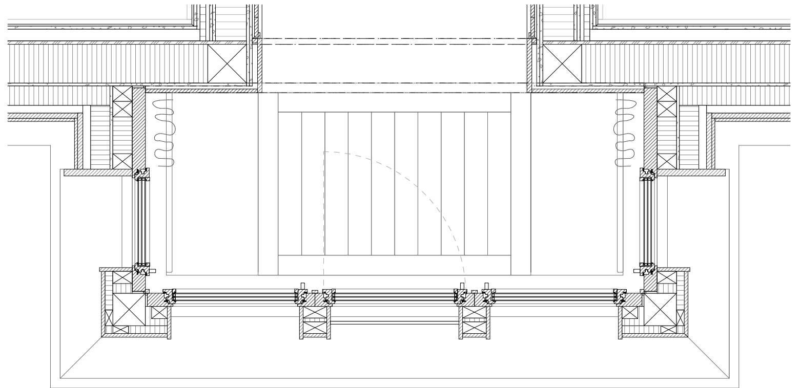
Grundriss
