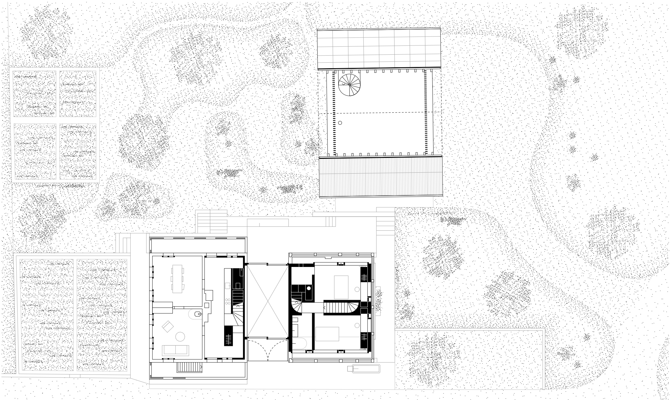
GRUNDRISS - OBERGESCHOSS
