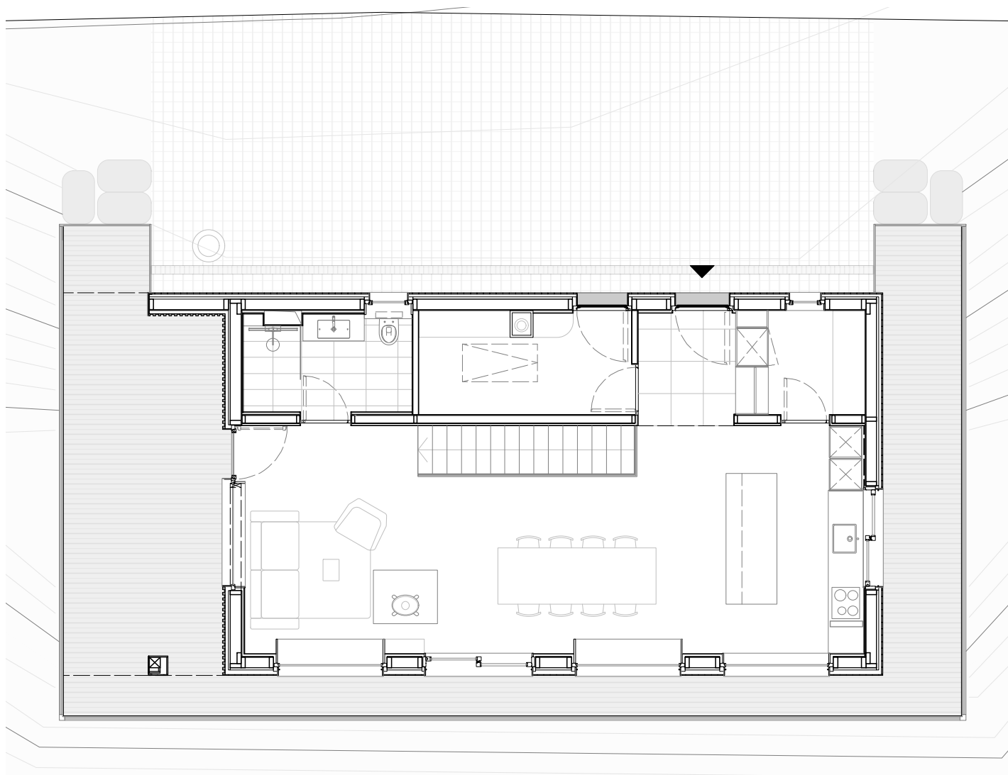
Plan rez-de-chaussée
