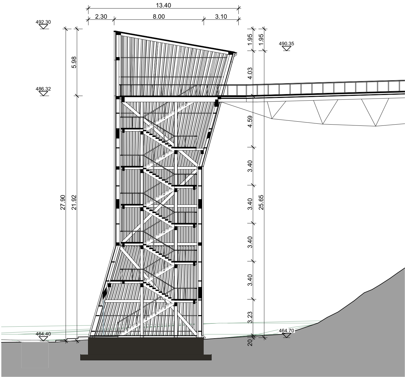
Längsschnitt S - S
