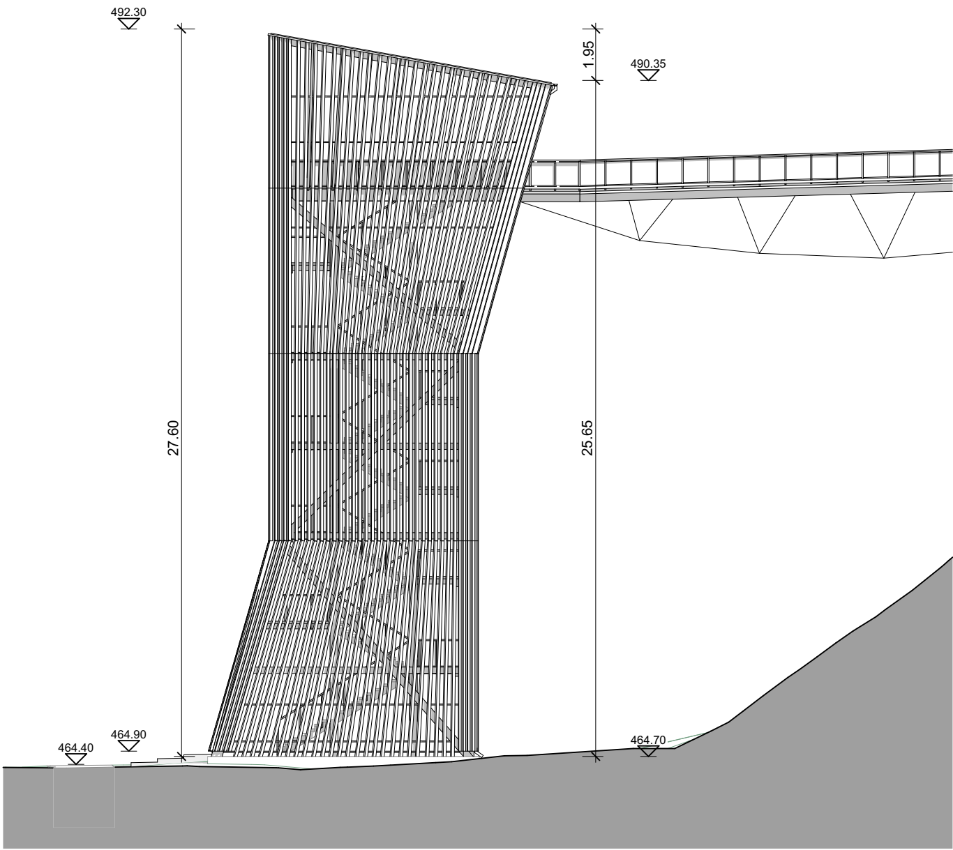
Ansicht West
