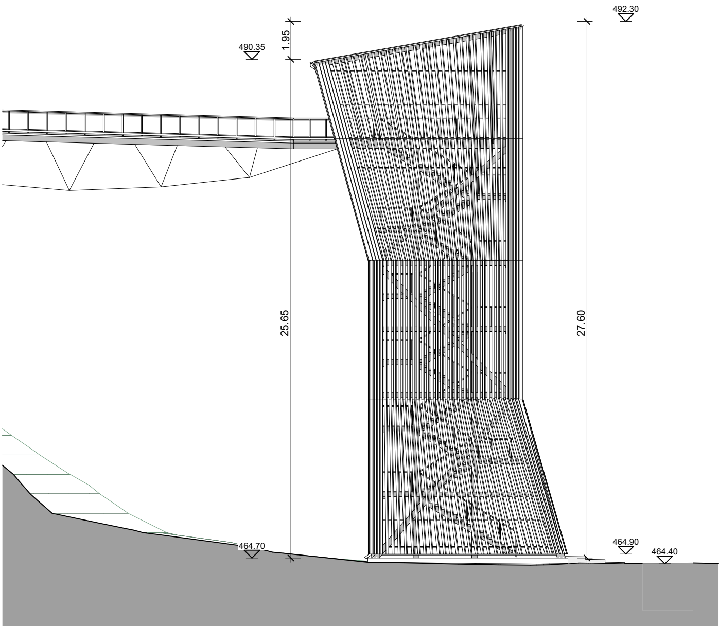
Ansicht Ost
