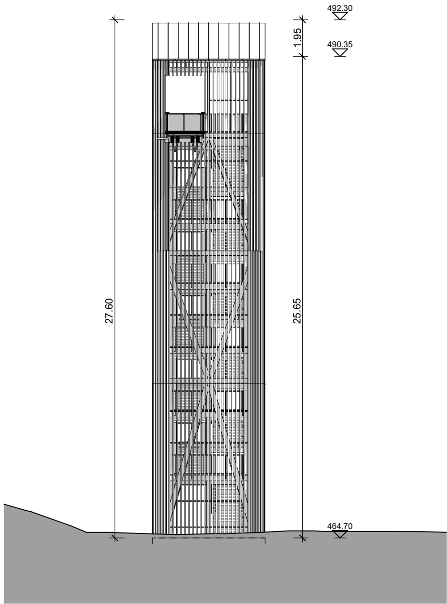
Ansicht Süd
