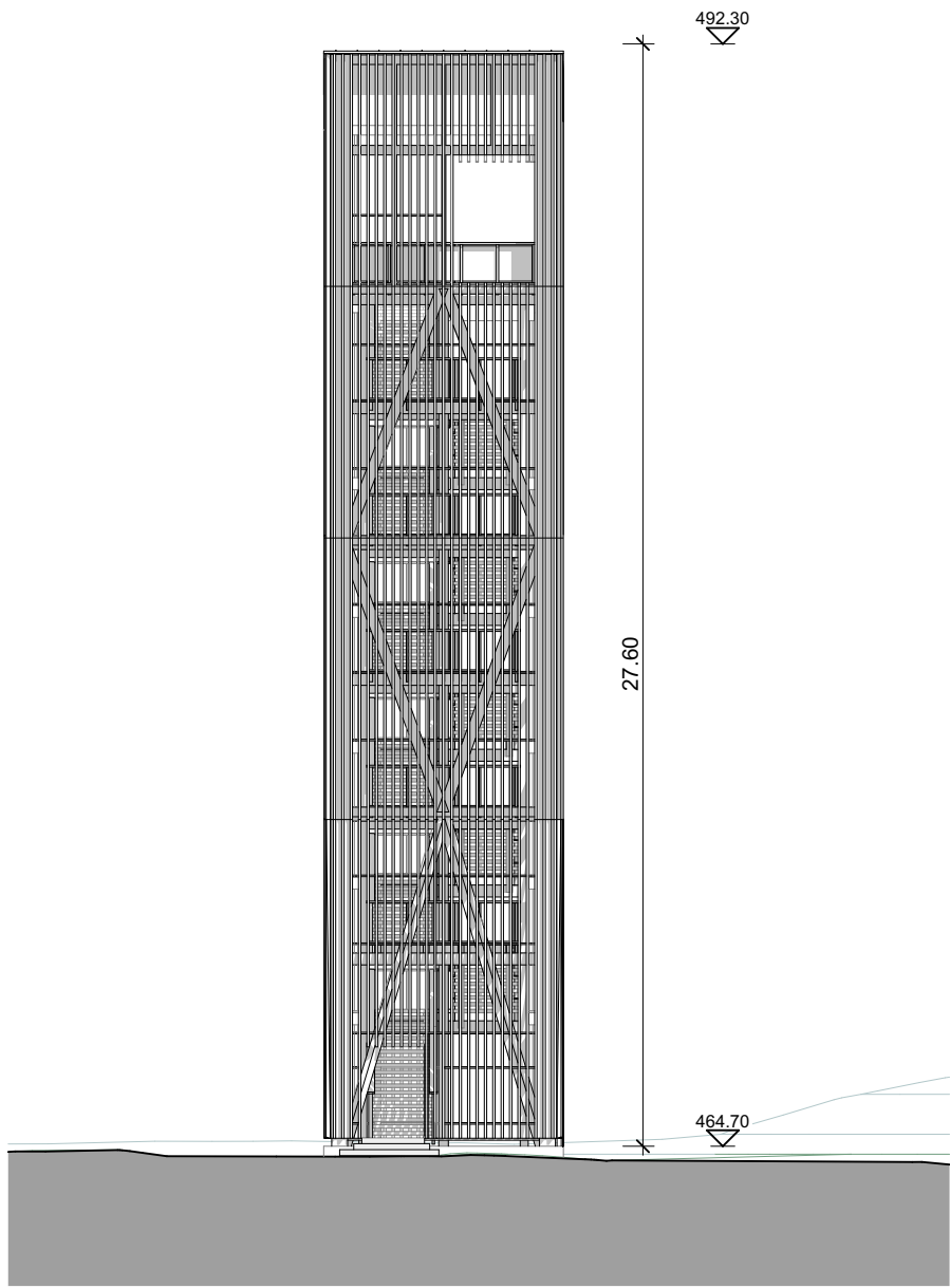
Ansicht Nord
