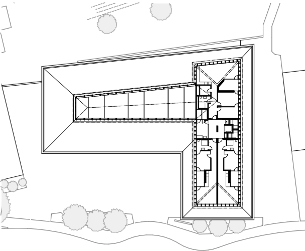
Dachgeschoss | Étage sous toiture
