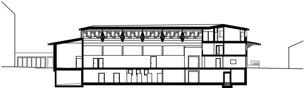
Schnitt B | Coupe B
