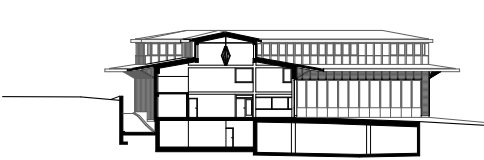
Schnitt A | Coupe A
