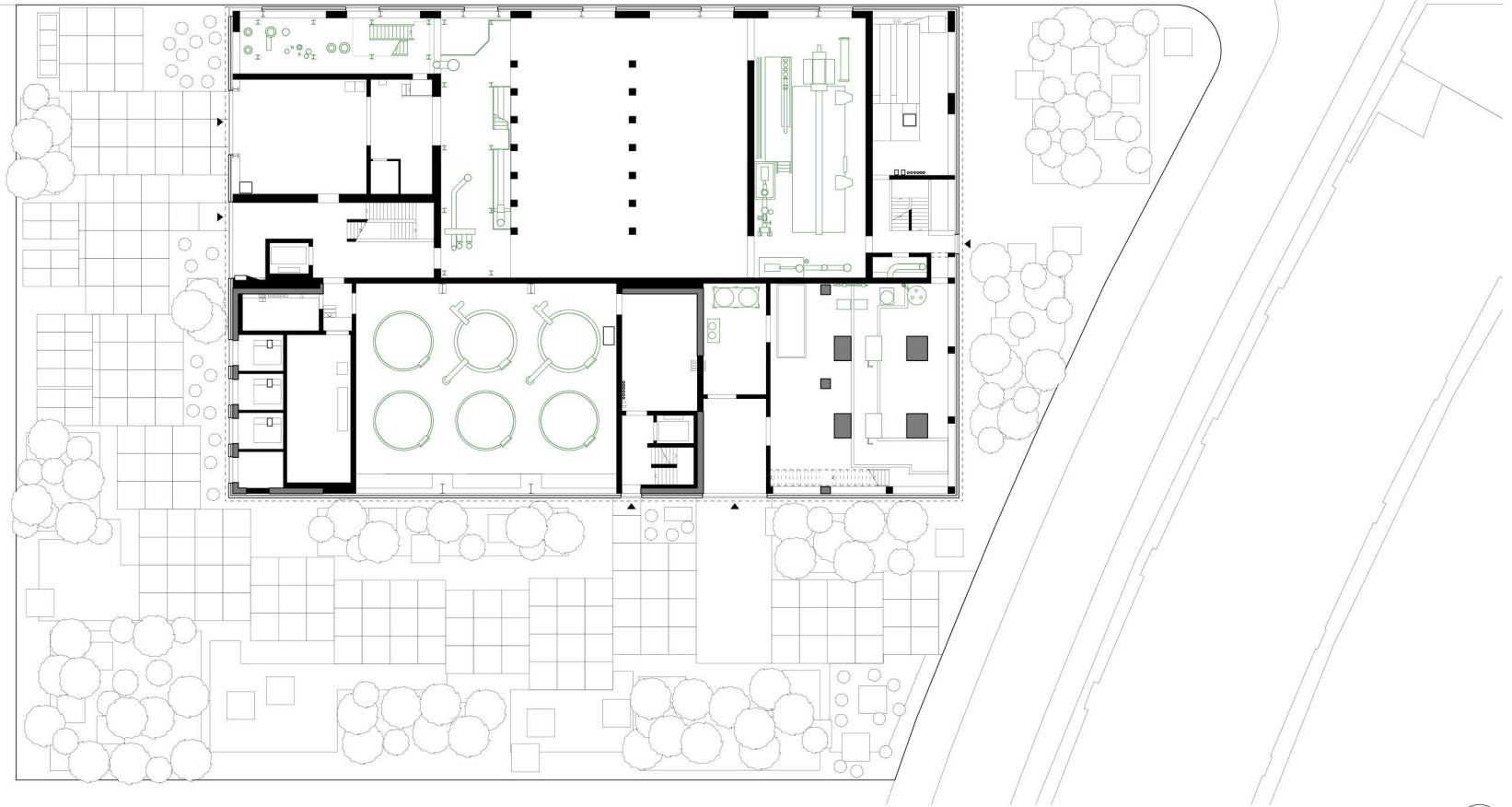
Grundriss Erdgeschoss, WZW Energiezentrale Josefstrasse, Zürich 1:500
