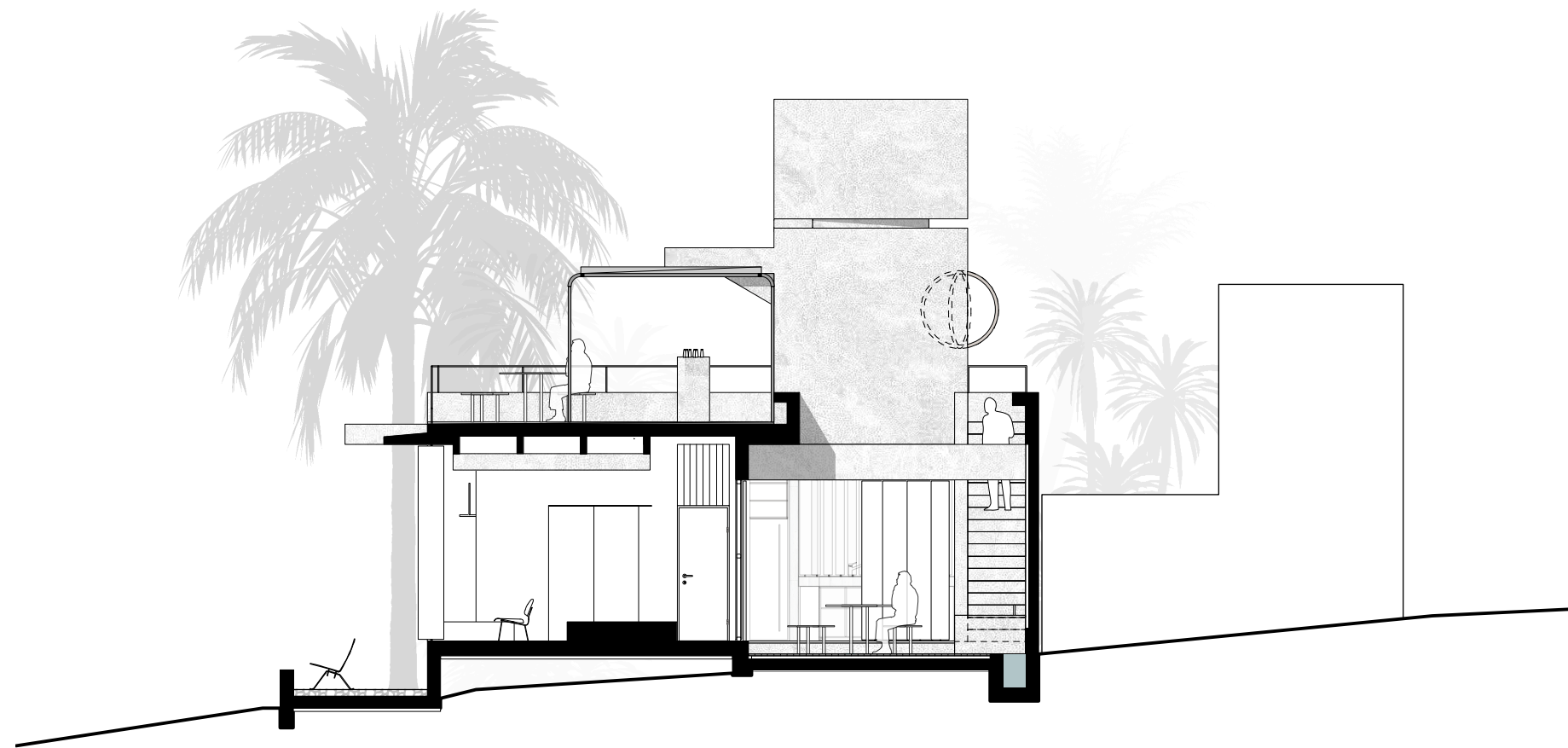
Schnitt C-C, Mst. 1:100
