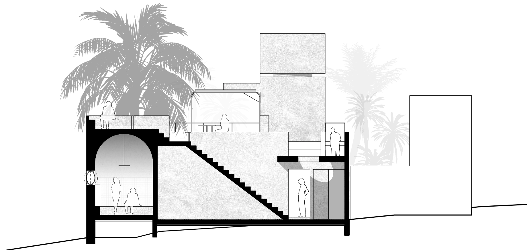
Schnitt D-D, Mst. 1:100
