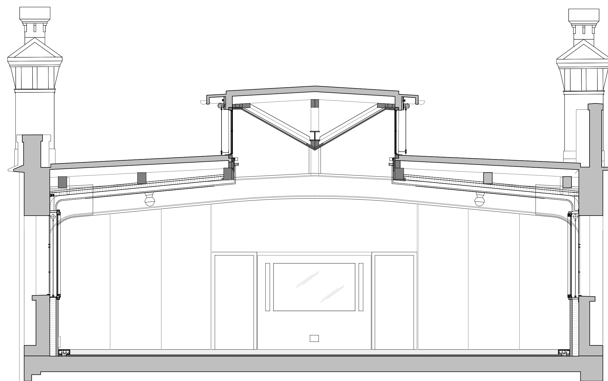
SCHNITT BLAUER SAAL RICHTUNG KÜCHE
