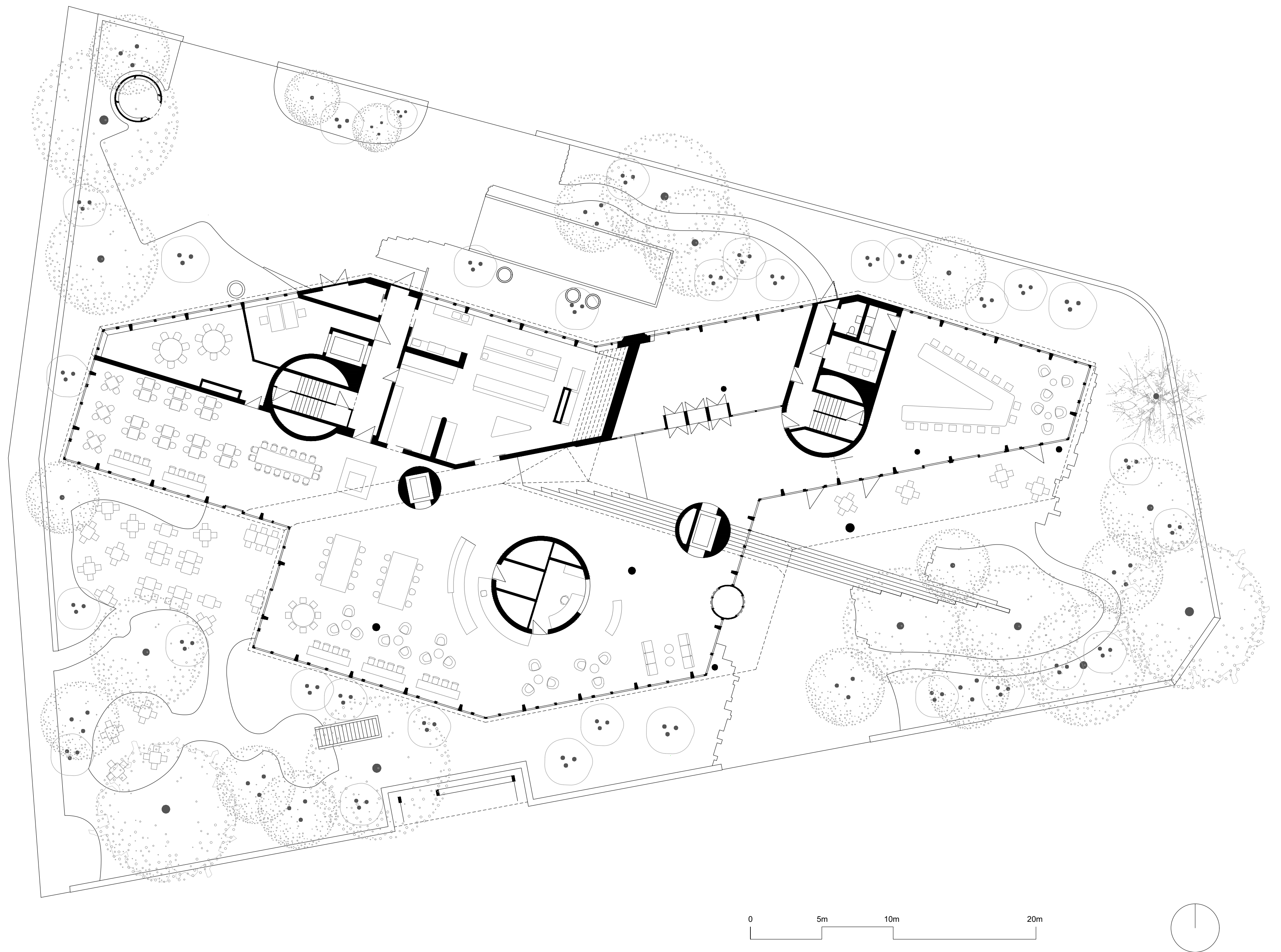
Erdgeschoss MST 1:200
