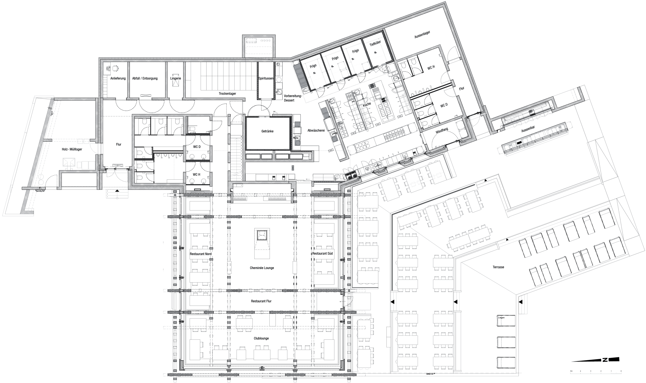
Grundriss Erdgeschoss
